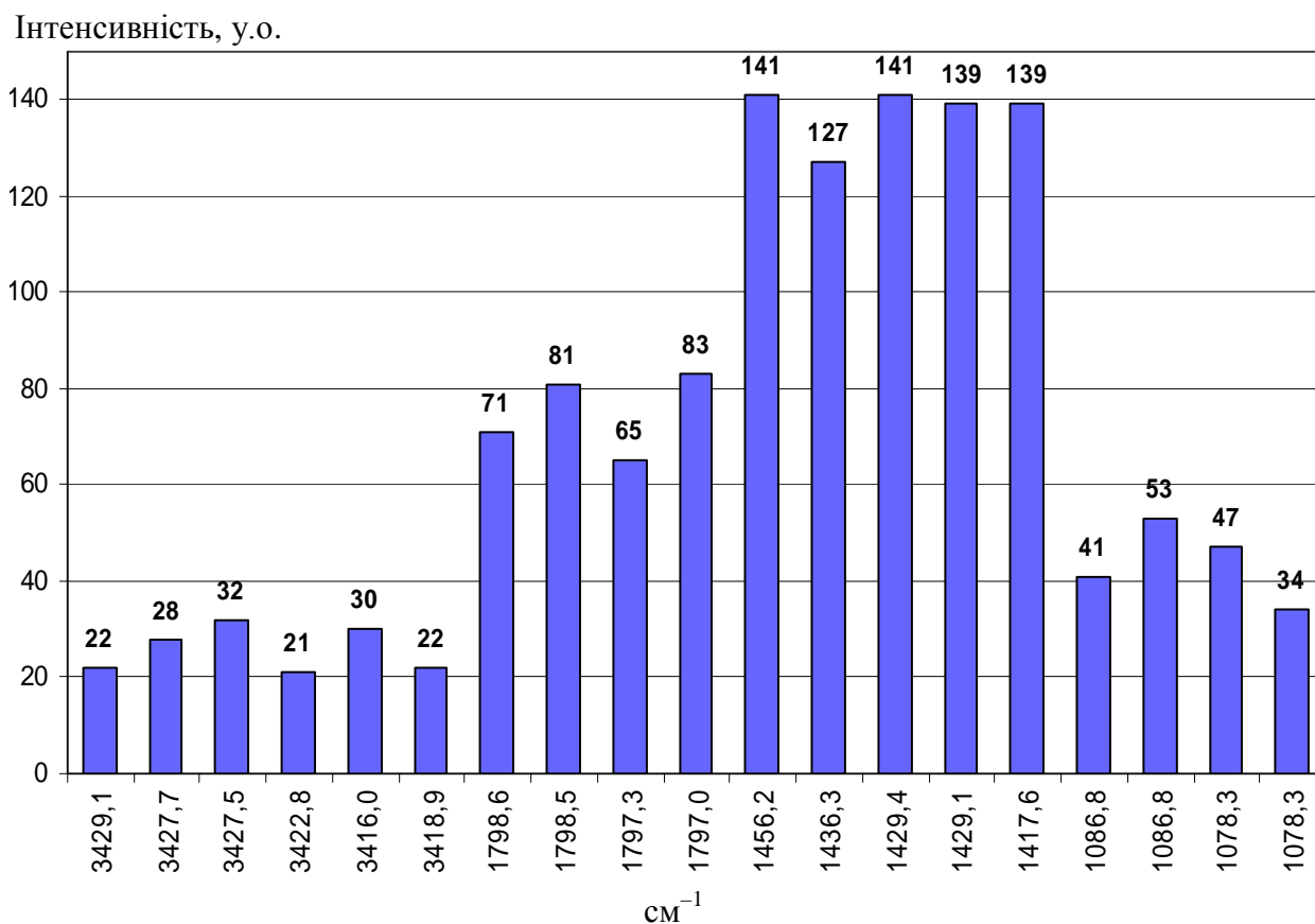
Рис. 2. Положення ( \text{cm}^{-1} ) та інтенсивність (у.о.) характеристичних смуг в ІЧ-спектрах вітчизняних і закордонних карбонатних наповнювачів:
