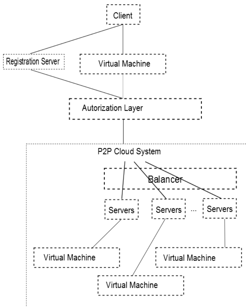
Рис. 1 – Архітектура відкритої хмарної системи
