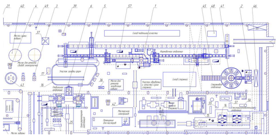
Рис.1 – Схема формовочного участка литейного цеха, подлежащего техническому перевооружению
