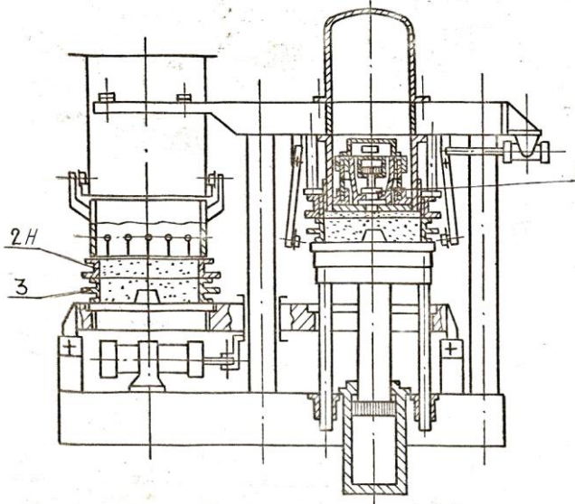
Рис. 6 – Подпрессовка
