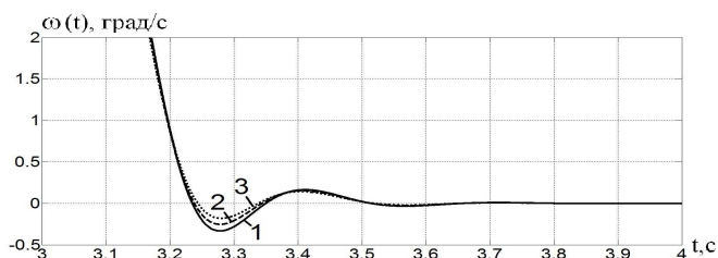
Рис. 5 - Перехідні процеси замкненої системи електрогідравлічного слідкуючого привода для вибраного значення 15 градусів для кутової швидкості об'єкту керування: 1 – штатний регулятор; 2 – регулятор з трикутною функцією приналежності; 3 – регулятор з використанням методу субтрактивної кластеризації
