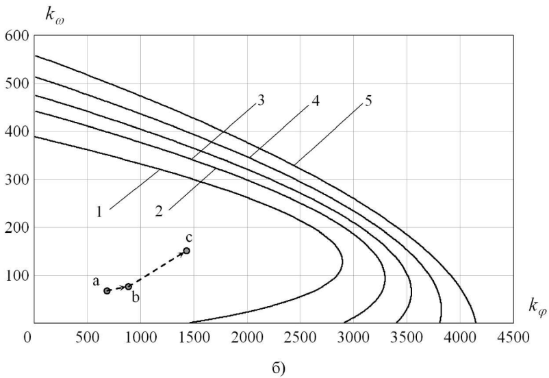
Рис. 2. Области стійкості замкненої системи наведення і стабілізації танкової башти з ЕМП (а) і ТПП (б):
