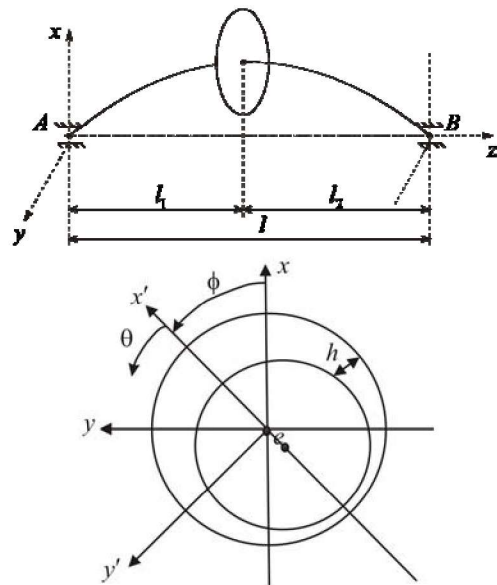
Рис.1. Расчетная схема однодискового ротора в подшипниках скольжения
