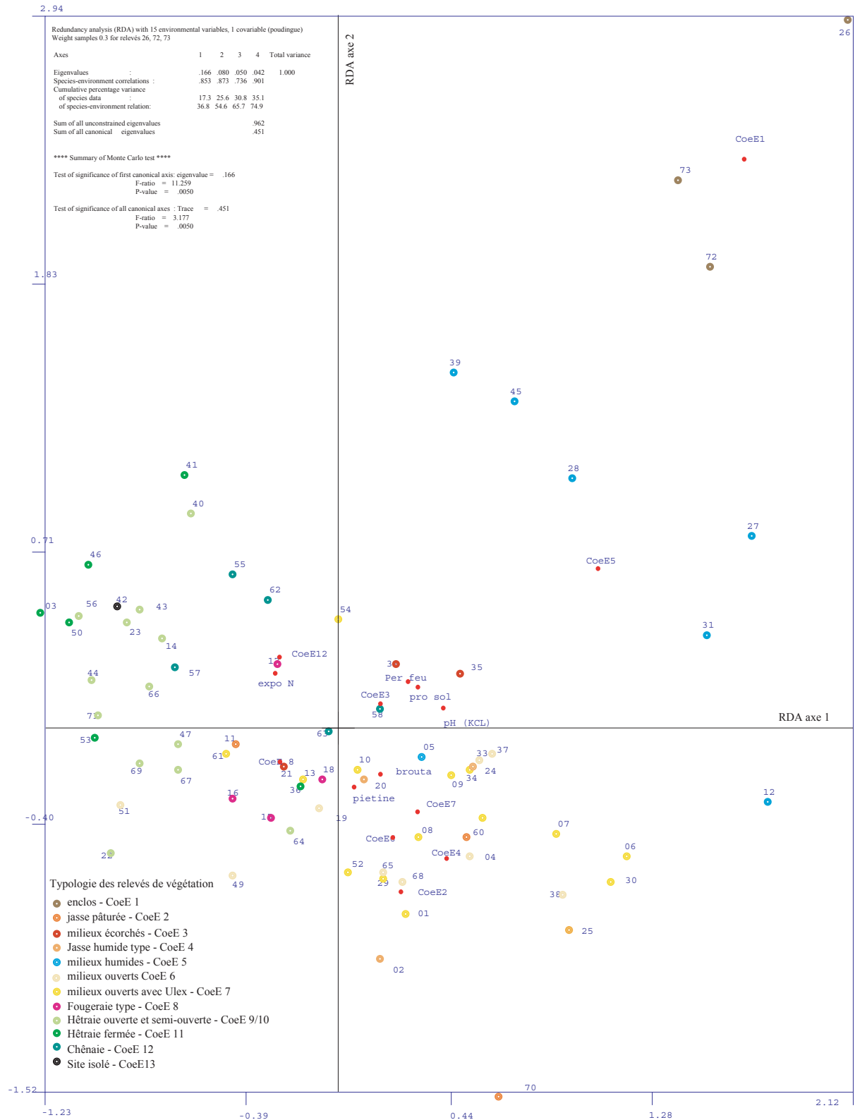
Fig.2. 4 : Analyse de redondance des spectres polliniques de surface. Calculs effectués à partir de la matrice 71 sites x 85 taxons et 71 sites x 37 variables explicatives. Forward selection de 15 variables et une covariable poudingue. Pondération 0.3 des échantillons 26, 72, 73. Représentation du plan des axes 1 et 2 des spectres polliniques actuels et des variables explicatives
