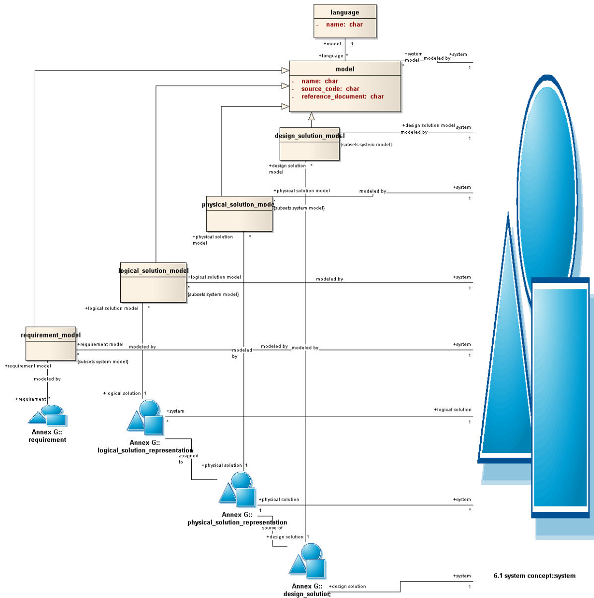
FIG. 4.12: Langues et système. Au cours de son développement, un système passe par plusieurs représentations : solution logique, solution physique et solution de conception. Un ou plusieurs modèles spécifiques sont associés à chacune de ces représentations ainsi qu'aux exigences du système. Ces modèles sont exprimés dans des langues dédiés.
