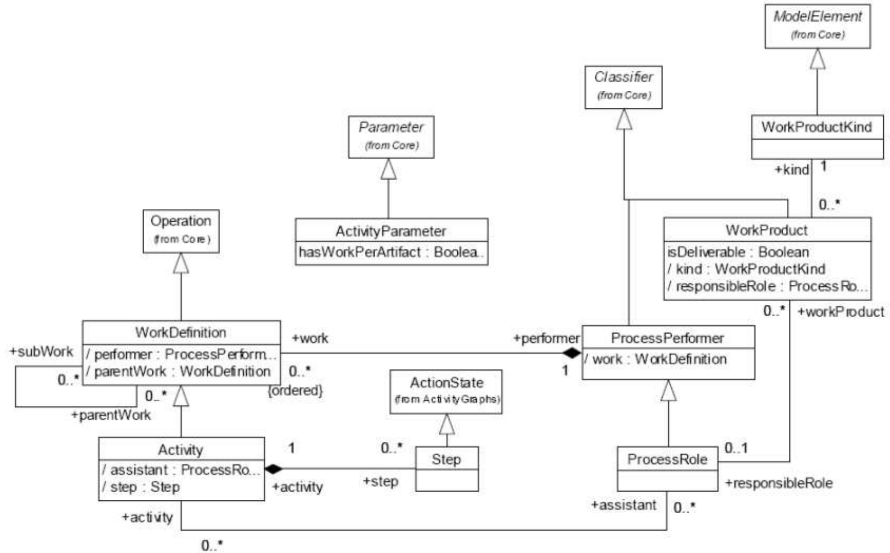
FIG. 2.6: Structure de processus en SPEM . Une représentation simplifiée de ce schéma est donnée figure 2.5. En plus des éléments déjà présentés sur ce dernier, on peut remarquer que les définitions de travail, i.e. les activités peuvent comprendre des sous-travaux. On peut imbriquer des activités les unes dans les autres. Les activités peuvent aussi comprendre des étapes qui correspondent à la plus petite unité de description des processus (figure 7-1 de [OMG05]).
