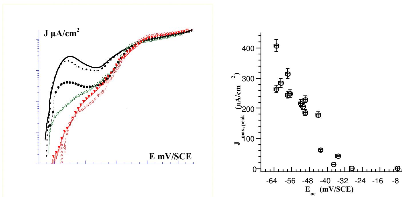
figure 11a : Cu-13Sn (%m.) en milieu aqueux \text{Na}_2\text{SO}_4 (0.01M) (RDE 1000 rpm) à gauche ) Courbes de polarisation anodique pour différentes valeurs de E_{\text{oc}} (B à E : temps d'immersion croissants) à droite ) Relation entre les densités de courant du pic anodique ( J_{\text{max,peak}} ) et E_{\text{oc}} .
