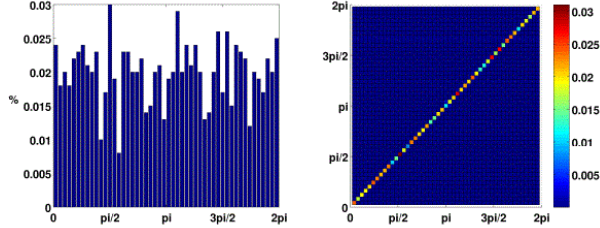
(d) N = 10^5
