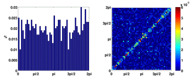
(d) N = 10^5
