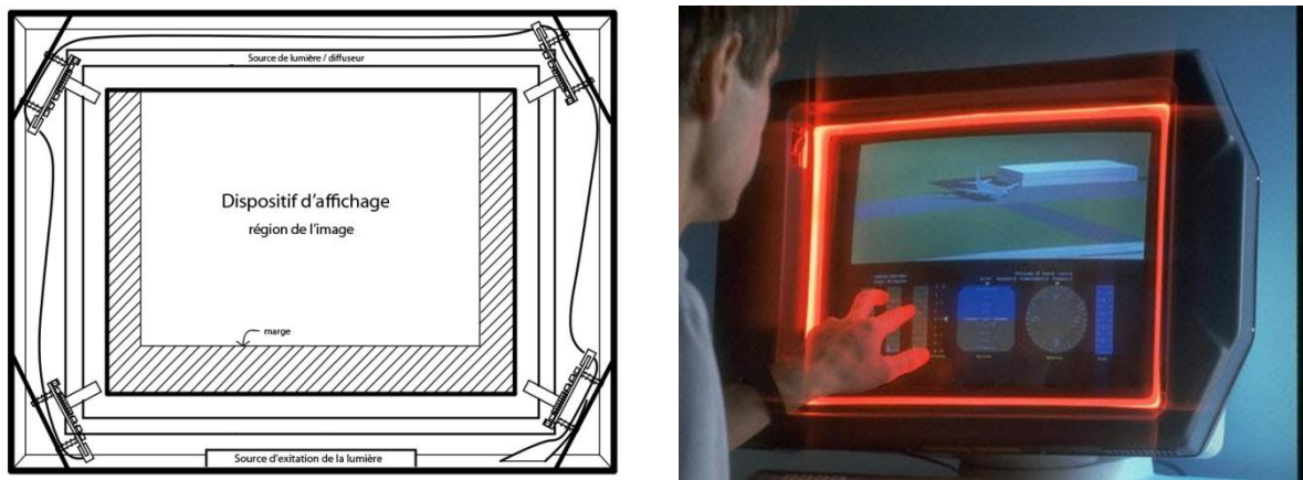
Figure 16 - SensorFrame . A gauche, schéma du dispositif, reproduction. A droite, photo du dispositif. In [McAviney Paul, 1986]
