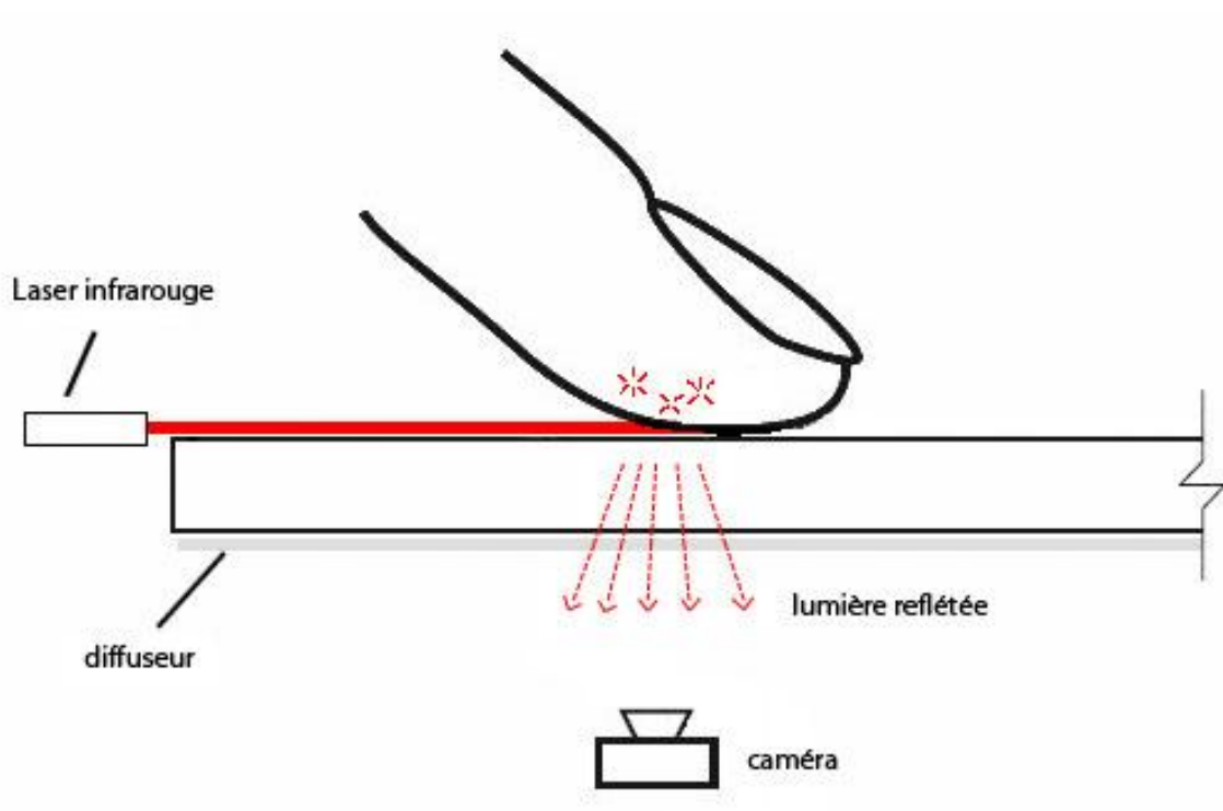
Figure 45 - Configuration d'un système LLP. Reproduction. In [SCHÖNING, 2008].
