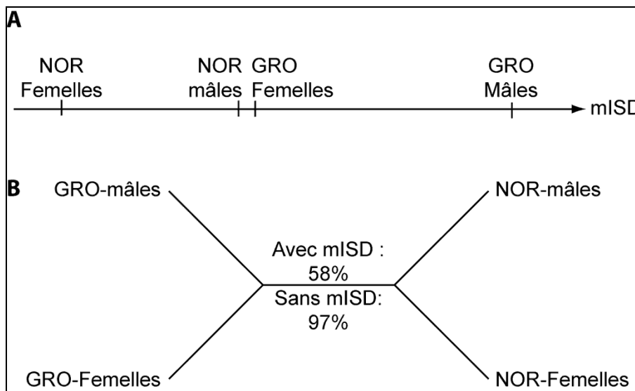
Figure 113 : Comparaison des deux sexes pour les écotypes de toundra (Groenland) et de montagne (Norvège) (indice VSI*, 33 variables) par analyse de groupement (méthode d'ajustement aux moindres carrés). A. Valeurs relatives de mISD calculées pour chaque échantillon, illustrant les différences de tailles isométriques entre écotypes et sexes ; B. Arbre obtenu à partir des valeurs de VSI* « brutes » et « centrées ». Les pourcentages sur la branche interne de l'arbre sont les valeurs de support bootstrap (10 000 itérations), indiquant la confiance statistique associée au regroupement par écotype des deux sexes.
