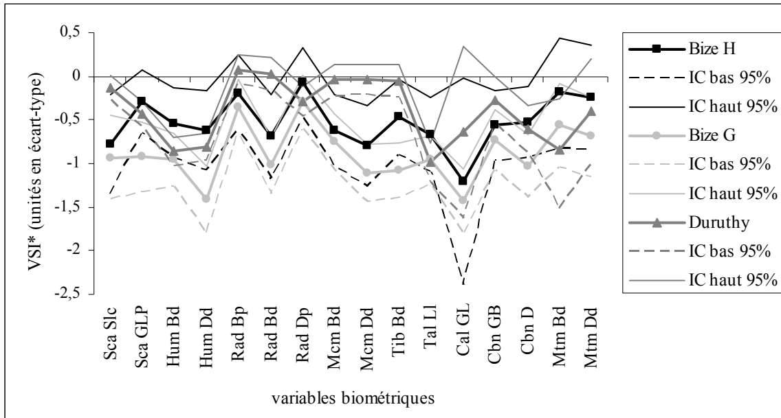
Figure 159 : Diagramme de Simpson montrant les différences entre Duruthy et Bize. Echantillon de référence : Stellmoor (VSI*= 0).
