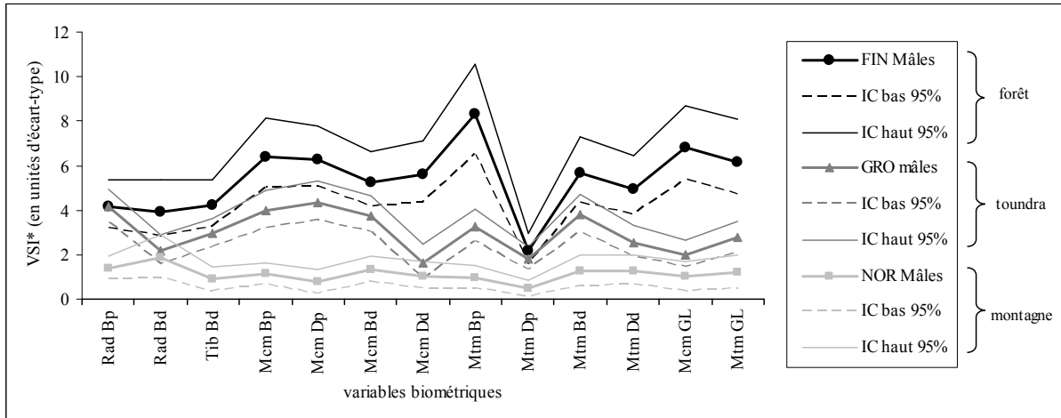
Figure 107 : Comparaison des mâles de forêt (Finlande), de toundra (Groenland) et de montagne (Norvège) (Indice VSI*). L'assemblage de mâles et de femelles de Norvège est utilisé comme référence ( VSI^* = 0 ). Les valeurs obtenues pour les trois échantillons diffèrent significativement ( p [H_0 : mISD_{FIN} = mISD_{GRO}, mISD_{FIN} = mISD_{NOR}, mISD_{GRO} = mISD_{NOR}] = 10^{-4} ).
