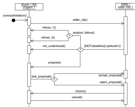
Figure 2.1 — Représentation d'un protocole d'interaction grâce à un diagramme de séquence A-UML.
