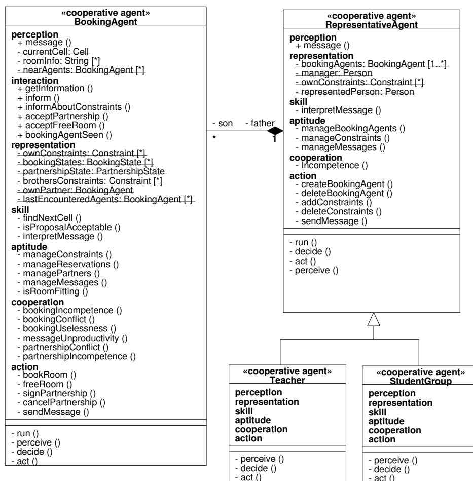
Figure 3.22 — Diagramme de classes d’agents pour ETTO.
