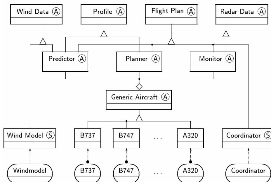
Figure 2.7 — Un exemple de diagramme de classes et d'instances pour le problème du trafic aérien dans AAI.
