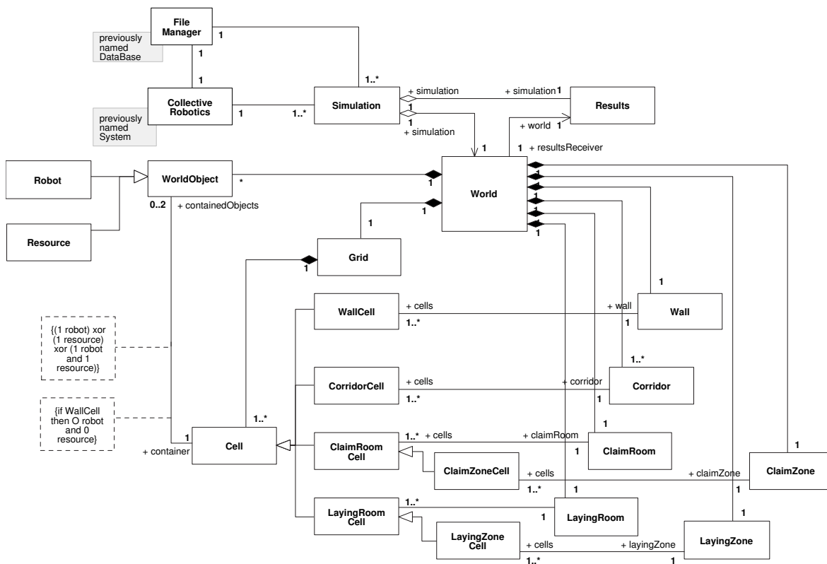
Figure 6.2 — Le diagramme de classes préliminaire d’analyse pour le problème de transport collectif.
