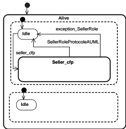
Figure 4.4 — Machine à états finis pour la classe Seller du protocole de la figure 4.1.
