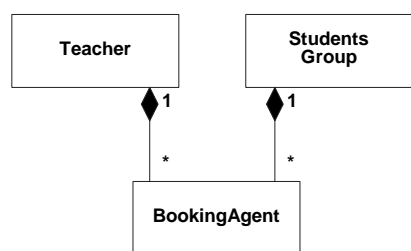
Figure 3.17 — Diagramme de classes du paquetage agent.
