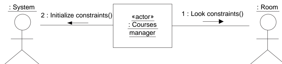
Figure 3.5 — Diagramme de collaboration entre le système et les salles.
