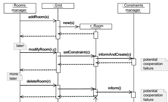
Figure 3.14 — Diagramme de séquences d'ETTO représentant les interactions entre le gestionnaire de salles et les salles.
