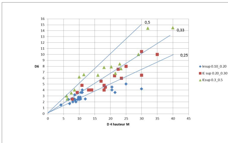
Figure 25 : répartition des formes de catégorie B et C selon l'indice IH = D6/D4 en fonction de l'indice d'élanement de la panse supérieure IEsup = D6/D3 .
