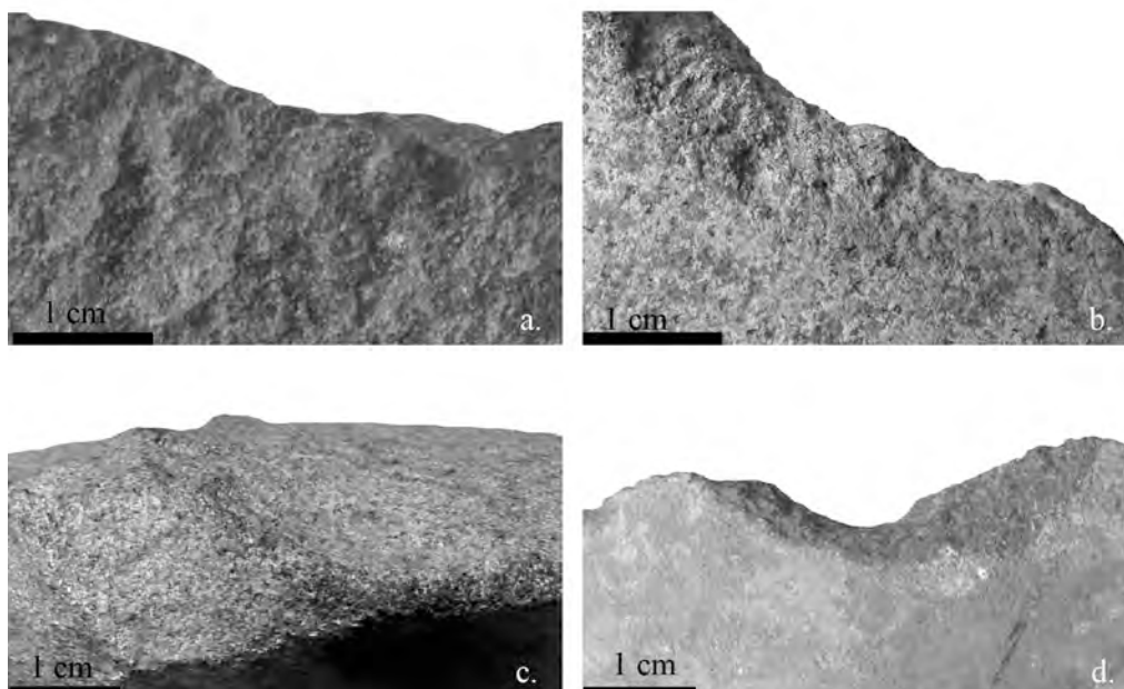
Fig. 69 : Exemples des états de surface des hachereaux d'Olha I. a : quartzite ; b : opiate altérée ; c : nervures émoussées ; d : esquillement récent (Photos et DAO : M. Deschamps).
