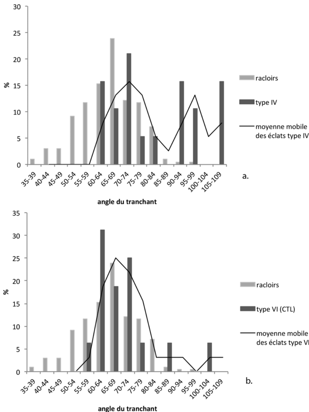
Fig. 378 : Olha II, histogramme des angles des tranchants des racloirs par classe de 5°, comparé aux : a. angles des tranchants antérieurs sur les éclats de type IV ; b. angles des tranchants antérieurs sur les coups de tranchets latéraux.
