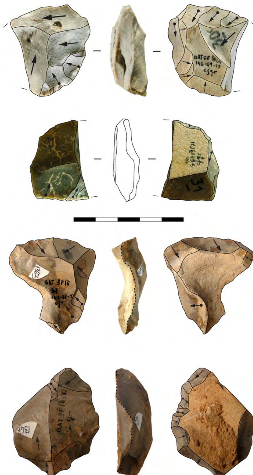
Fig. 321 : Gatzarria-Cjr, nucléus et fragments de nucléus en silex présentant un haut degré d'exhaustion : a et b : nucléus fracturés ; c et d : nucléus présentant un dernier enlèvement envahissant outrepassé.
