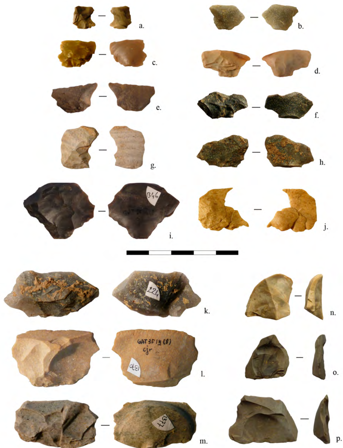
Fig. 334 : a. à i. : éclats de retouche en différentes matières premières ; j. : remontage de trois éclats de retouches ; k. à m. : éclats de ravigage ; n. à p. : éclat d'encoche (Photos et DAO : M. Deschamps).
