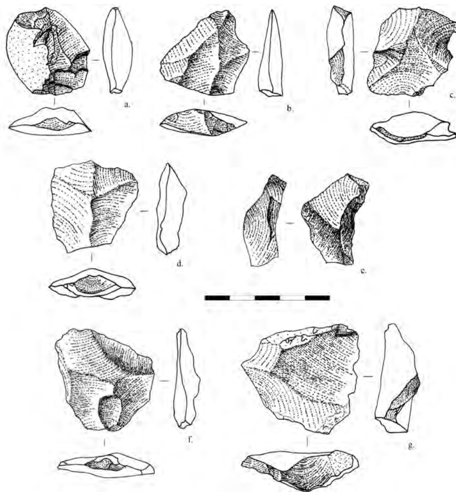
Fig. 365 : Olha II, éclats de débitage en quartzite : a : éclat cortical ; b à d : éclats ordinaires ; e : éclats à crête axiale ; f et g : pointe pseudo-Levallois (Dessins : M. Deschamps).
