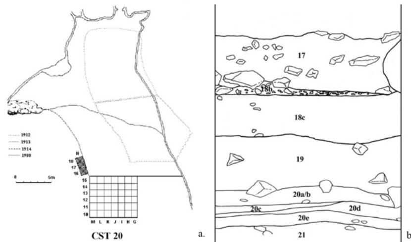
Fig. 37 : a : Plan des différentes fouilles ayant eu lieu à la grotte du Castillo (Cabrera, 1984) ; b : stratigraphie des niveaux 18 à 21 (Cabrera et al. 2001)
