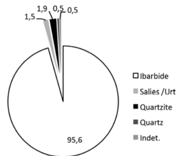
Fig. 156 : Pourcentage des matières premières hors matériel de percussion du niveau 25.
