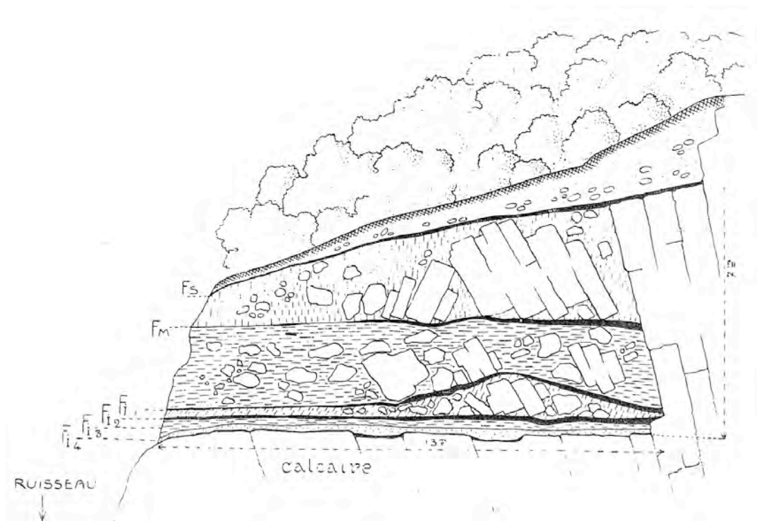
Fig. 338 : Coupe stratigraphique de l'abri Olha I (Passemar, 1936)
