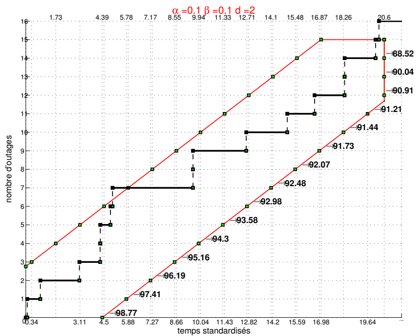
FIGURE 6 – Plan du test séquentiel pour un localiser de catégorie II avec \theta_1 = 2000 heures.
