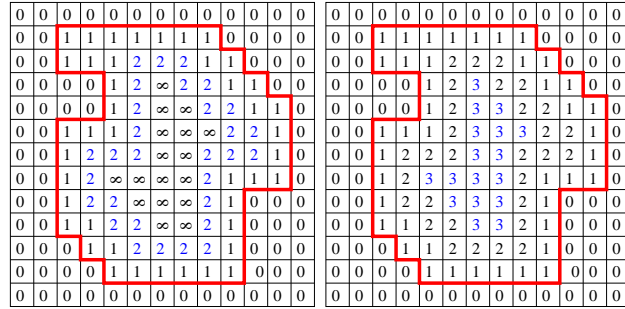
(d) first propagation (e) second propagation
