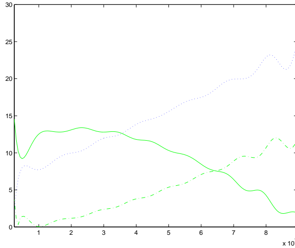
FIG. 21 – Erreur relative en pourcentage sur la transformée de Fourier du courant en module en fonction de la fréquence pour les différents modèles (...: Holl_1 , -: Fict_1 ; -.: Fict_{1,corr} )
