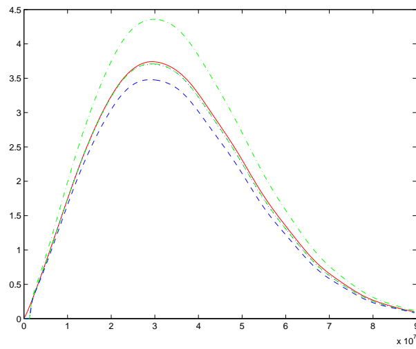
FIG. 14 – Module de la transformée de Fourier de la dérivée du courant en fonction de la fréquence pour les différents modèles (- : valeur statique, ... : Holl_{corr} et Fict_{corr} , - - : Holl_2 , - . : Fict_1 )
