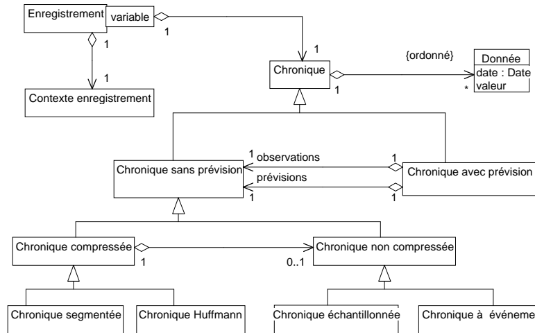
Figure 5 : diagramme de classes des enregistrements et des chroniques (notation UML, cf. annexe)
