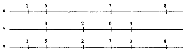
Figure III.4 : Exemple de diagramme temporel de l'instruction x:=u \text{ default } v , x, u et v sont de types entiers
