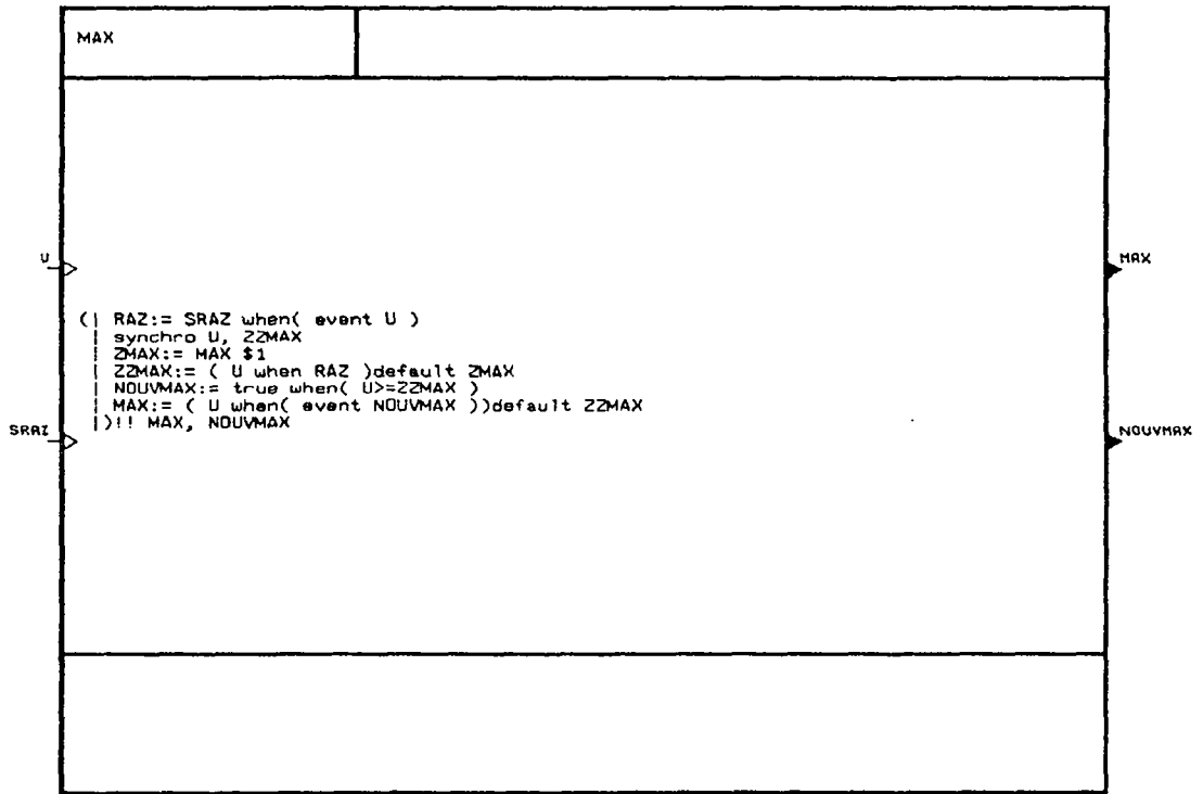
Figure A.9 : Le processus MAX
