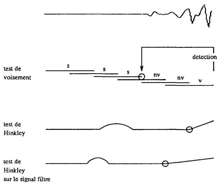
Figure IV.6 : La frontière détectée par le test de voisement est validée. Les étiquettes de voisement sont "s" pour silence, "v" pour voisé et "nv" pour non voisé.
