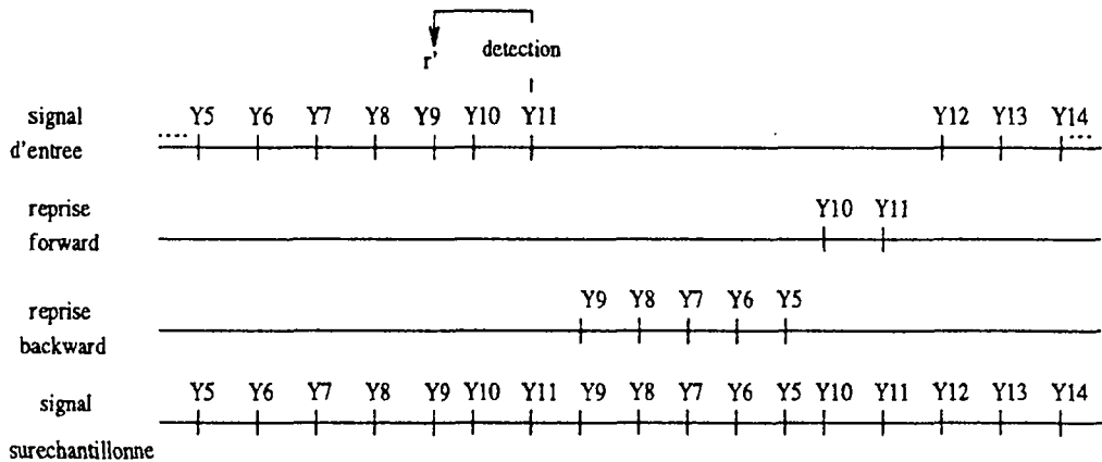
Figure IV.2 : Retour-arrière: une frontière est détectée à l'arrivée de l'échantillon Y11, la frontière étant localisée en Y9. Il y a un retour-arrière. La frontière n'est donc pas validée. On réinjecte les échantillons dans le sens rétrograde jusqu'à la dernière frontière (dans notre cas Y9 Y8 Y7 Y6 Y5, la dernière frontière est supposée placée en Y4). Le retour-arrière n'ayant rien détecté, la frontière est validée et placée en Y9. Il faut donc redémarrer à cette frontière et réinjecter les échantillons arrivés après Y9 (dans notre cas Y10 et Y11).
