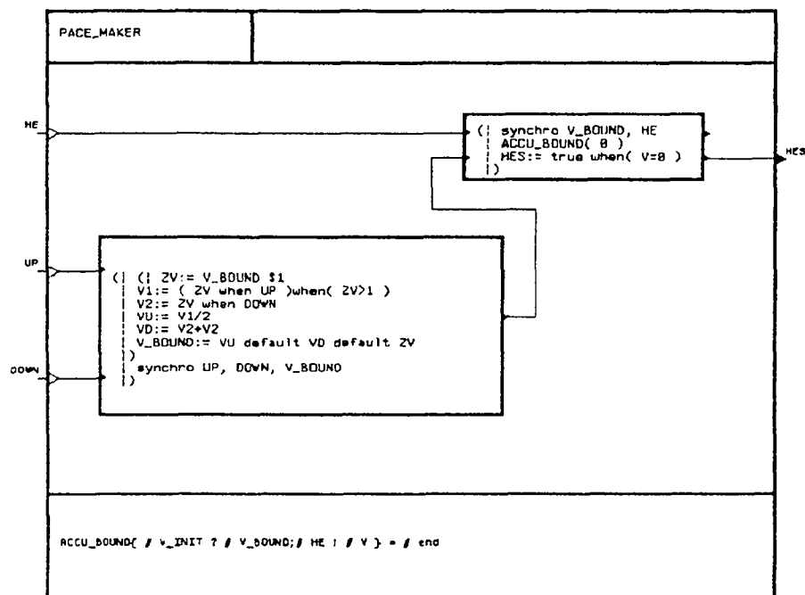
Figure V.4 : Le processus PACE_MAKER .
