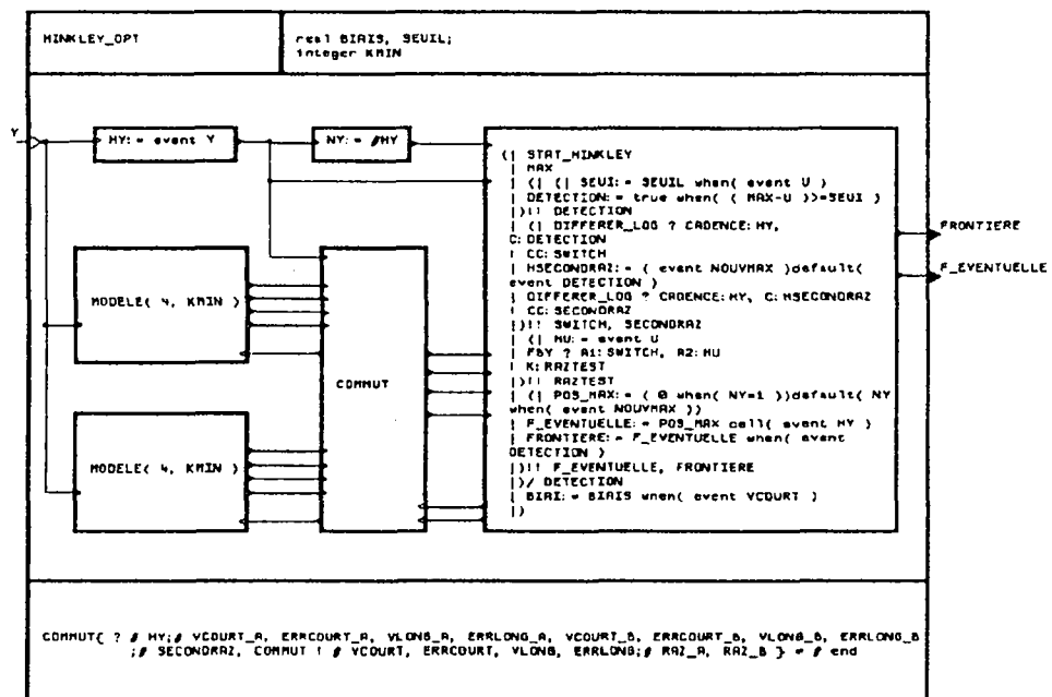
Figure IV.10 : Le processus HINKLEY_OPT
