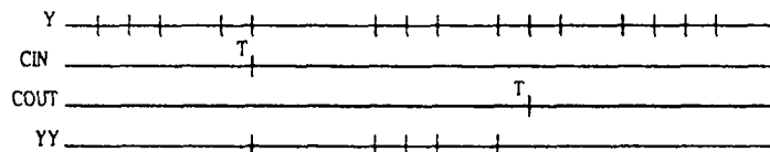
Figure B.13 : Exemple d'entrelacements des signaux du processus INTERRUPT
