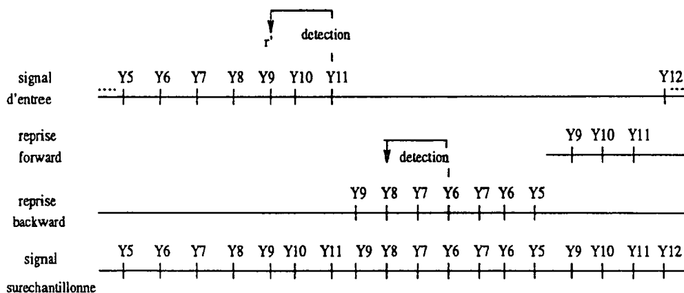
Figure IV.3 : Retour-arrière: une frontière est détectée à l'arrivée de l'échantillon Y11, la frontière étant localisée en Y9. Il y a un retour-arrière. La frontière n'est donc pas validée. On réinjecte les échantillons dans le sens rétrograde jusqu'à la dernière frontière (dans notre cas Y9 Y8 Y7 Y6 Y5, la dernière frontière est supposée placée en Y4). Une frontière est détectée à l'instant Y6 et localisée en Y8 pendant le retour-arrière. On met en attente cette frontière située en Y8. Et on redémarre le retour-arrière en Y8 (d'où la réinjection de Y7 et Y6 pendant le retour-arrière). A la fin du retour-arrière, la frontière située en Y8 est validée. Le redémarrage a lieu en Y8 (réinjection forward de Y9 Y10 Y11).
