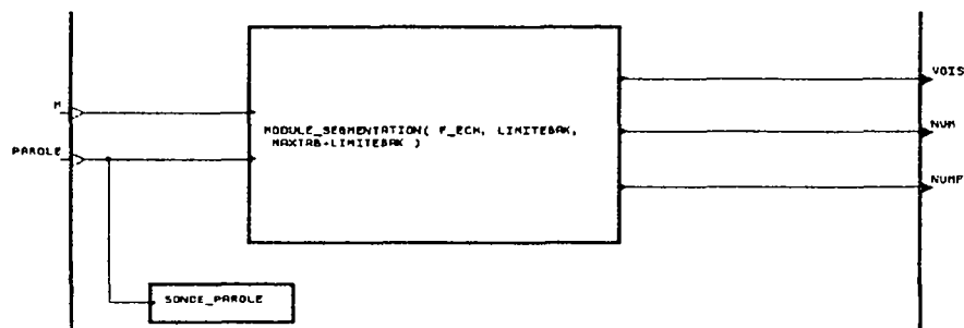
Figure V.1 : Le processus SONDE_PAROLE est associé au signal de parole.
