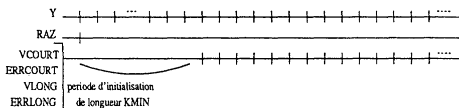
Figure IV.9 : L'entrelacement de signaux du processus MODELE
