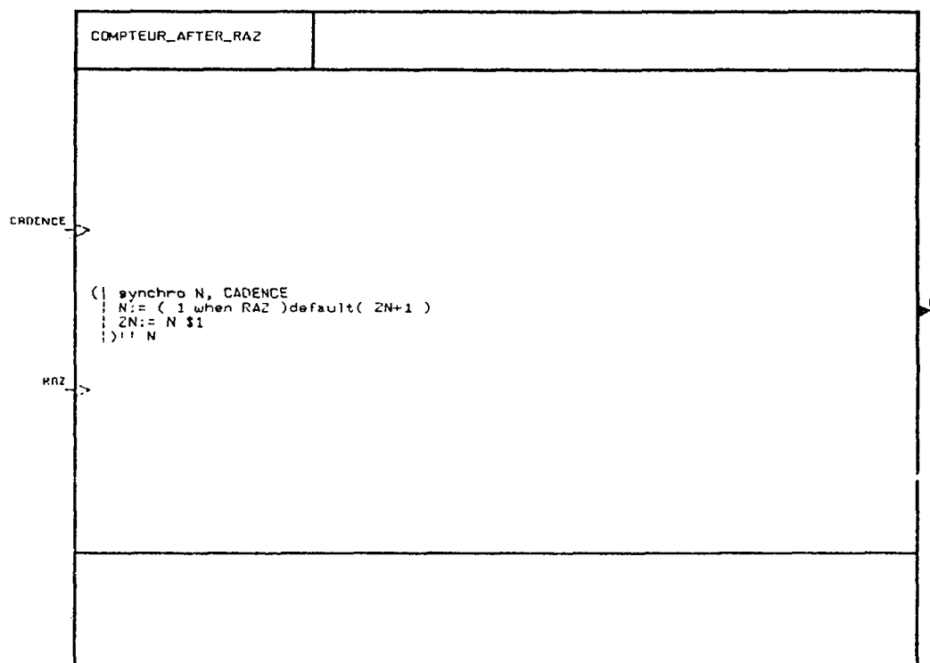
Figure B.3 : Le processus COMPTEUR_AFTER_RAZ
