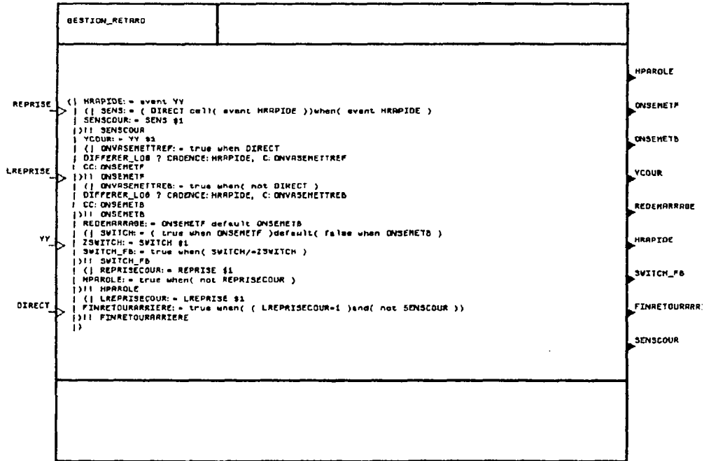
Figure IV.16 : Le processus GESTION_RETARD
