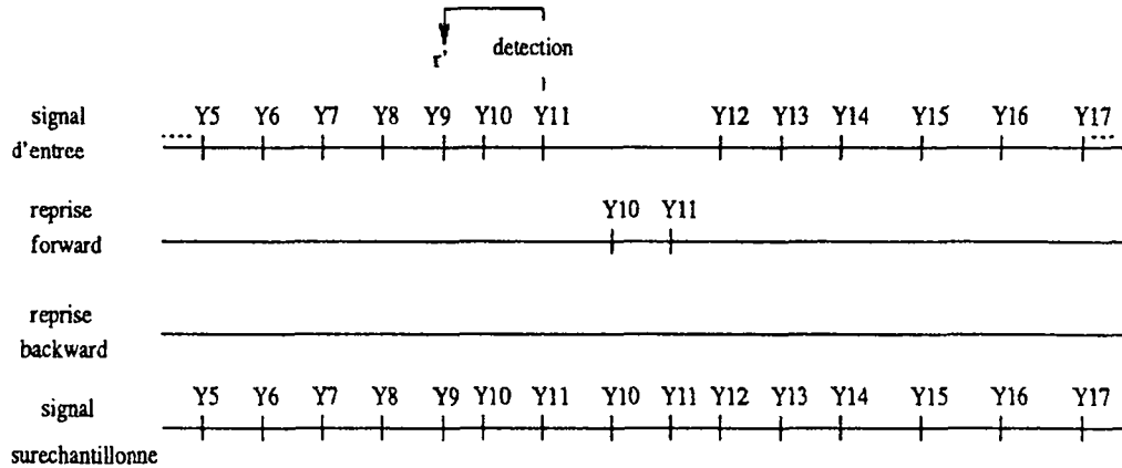
Figure IV.1 : Pas de retour-arrière: une frontière est détectée à l'arrivée de l'échantillon Y11, la frontière étant localisée en Y9. Il n'y a pas de retour-arrière. La frontière est donc placée en Y9 et il faut réinjecter les échantillons arrivés après Y9 (dans notre cas Y10 et Y11).
