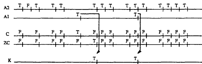
Figure B.11 : Exemple d'entrelacements des signaux du processus FBY
