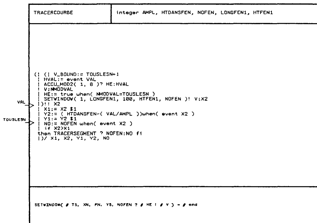
Figure C.3 : Le processus TRACERCOURBE
