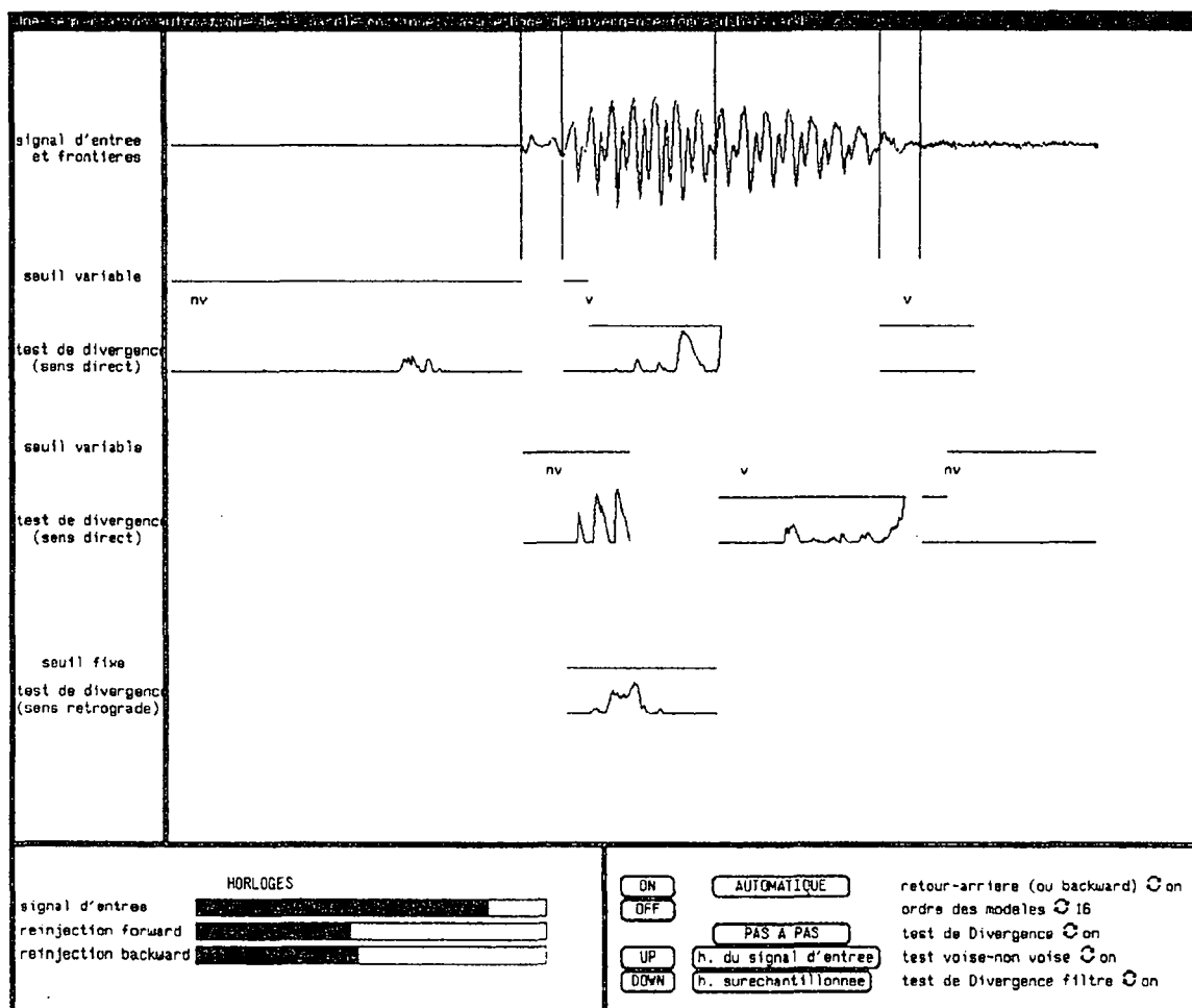
Figure V.10 : Environnement synchrone autour d'un module de segmentation.
