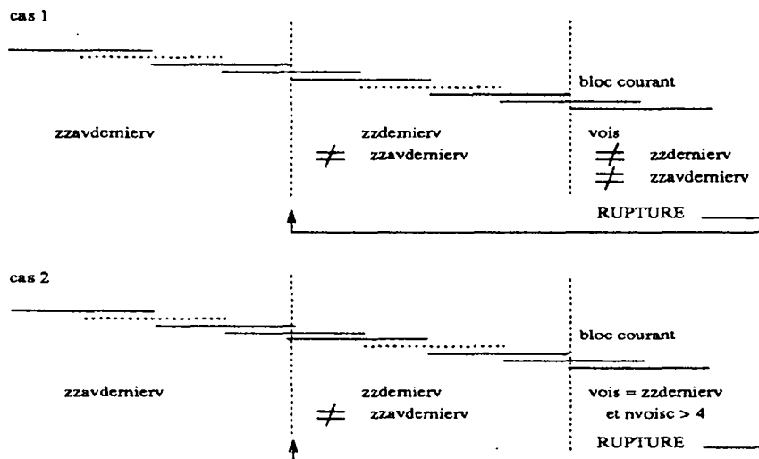
Figure IV.21 : La détection de frontières par le test de voisement. NVOISC est le nombre de blocs où la décision de voisement vaut ZZDERNIERV . Tous ces signaux sont synchrones à WY (test actif).
