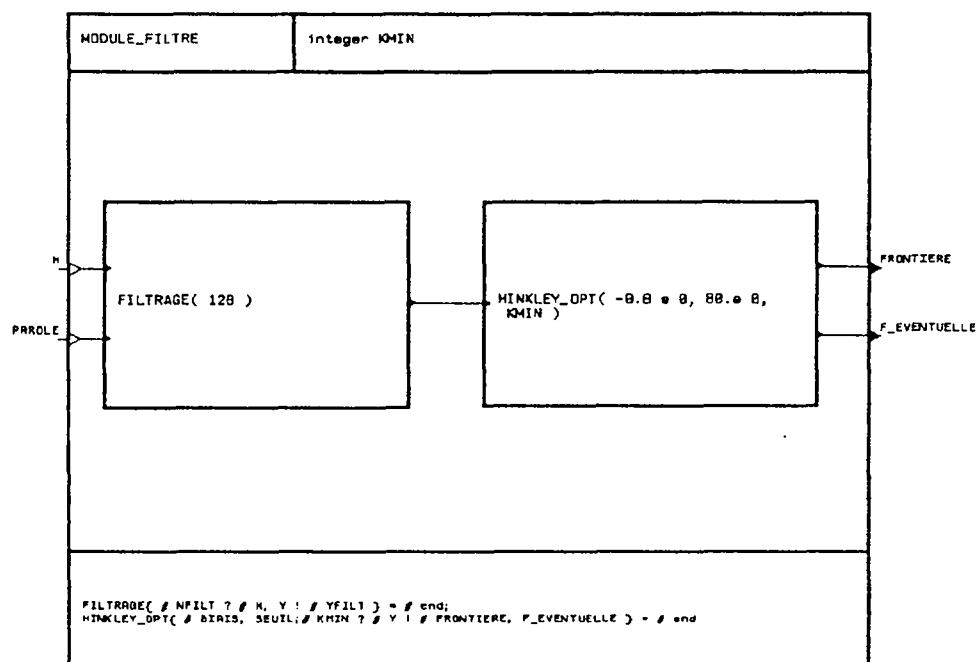
Figure IV.12 : Le processus MODULE_FILTRE
