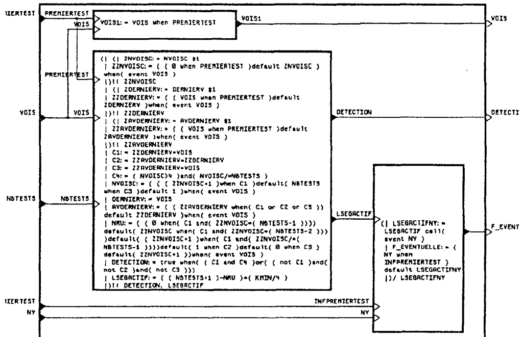
Figure IV.20 : La décision de voisement et la détection de frontières. Cette boîte noire est représentée de façon textuelle sur la figure IV.18.
