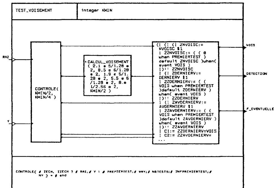
Figure IV.18 : Le processus TEST_VOISEMENT
