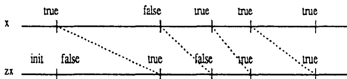
Figure III.5 : Exemple de diagramme temporel de l'instruction zx:=x \$ 1 , x et zx sont de types booléens
