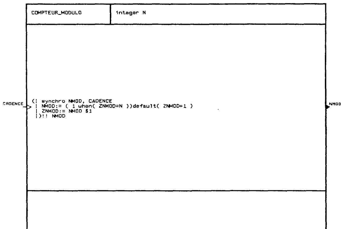
Figure B.4 : Le processus COMPTEUR_MODULO
