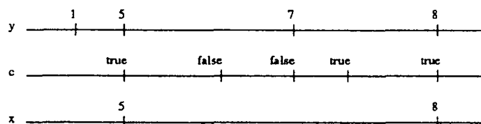
Figure III.3 : Exemple de diagramme temporel de l'instruction x := y \text{ when } c , x et y sont de types entiers
