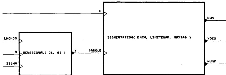
Figure V.6 : L'entrée PAROLE est générée par GENESIGNAL .
