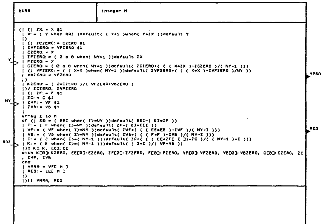
Figure A.5 : Le processus BURG
