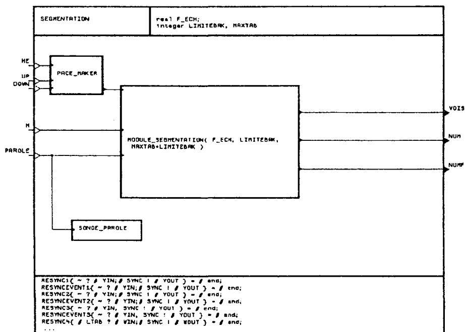
Figure V.5 : Une utilisation du PACE_MAKER .
