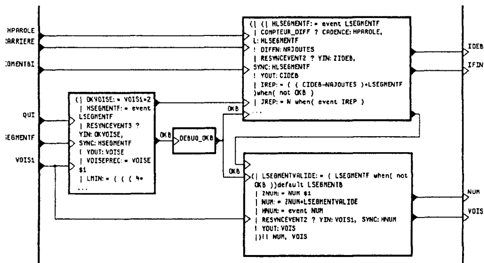
Figure V.3 : Le processus DEBUG_OKB est positionné entre le port diffuseur OKB et le port récepteur du lien. Cette figure représente un gros plan du processus GESTION_INDICES déjà présenté.
