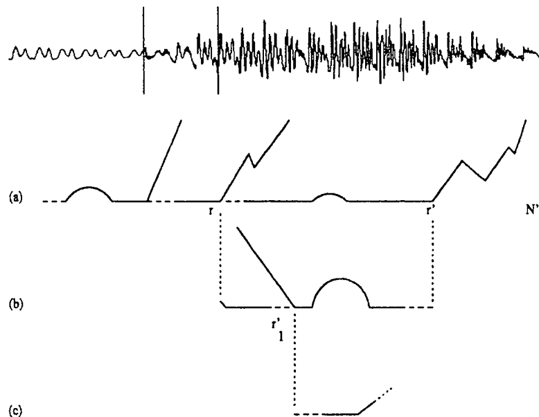
Figure II.4 : Le retour-arrière.
