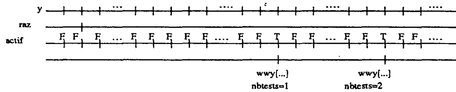
Figure IV.19 : L'entrelacement de signaux du processus CONTROLE
