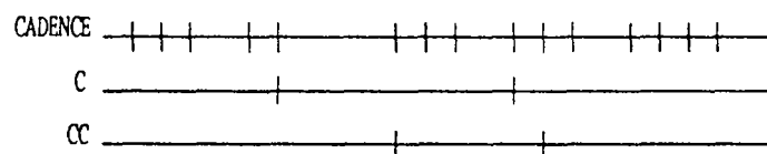
Figure B.15 : Exemple d'entrelacements des signaux du processus DIFFERER
