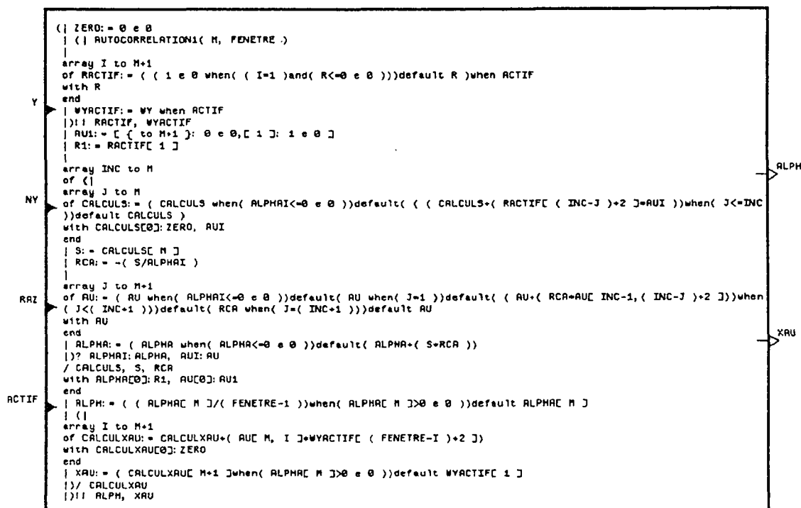
Figure A.4 : Le processus AUTO
