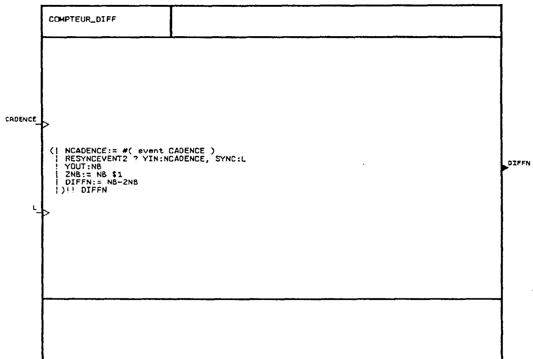
Figure B.8 : Le processus COMPTEUR_DIFF
