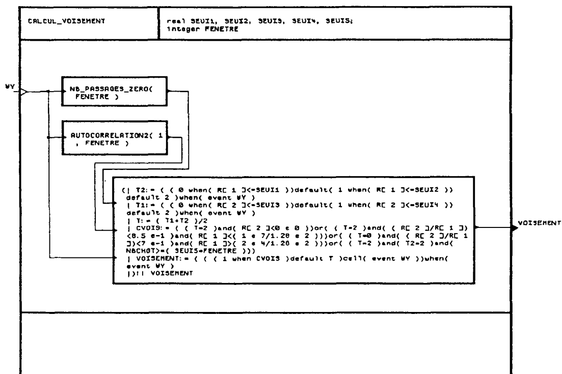
Figure A.10 : Le processus CALCUL_VOISEMENT
