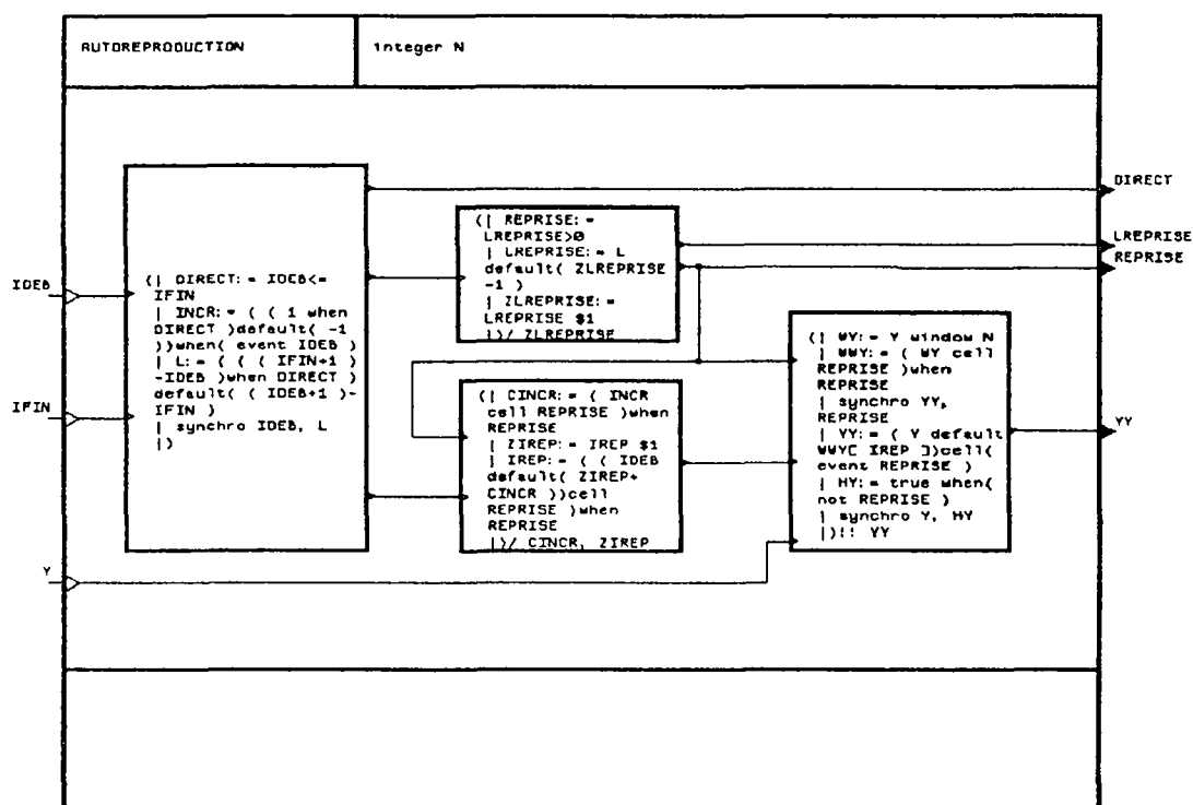
Figure B.16 : Le processus AUTOREPRODUCTION
