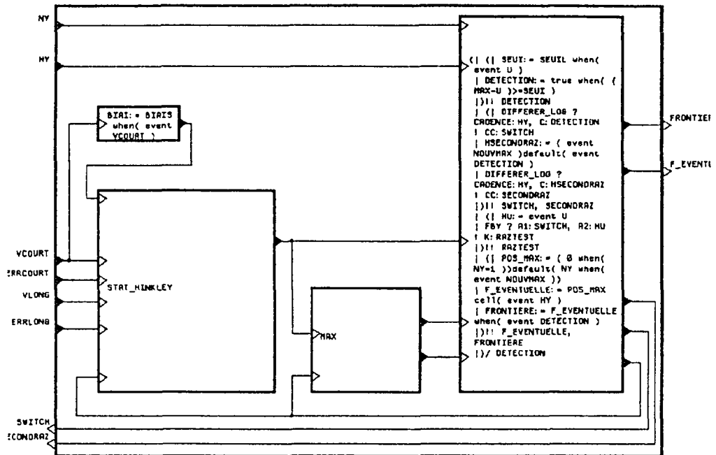
Figure IV.11 : Les trois phases effectuées par le processus primaire. Cette boîte noire est représentée de façon textuelle sur la figure IV.10.
