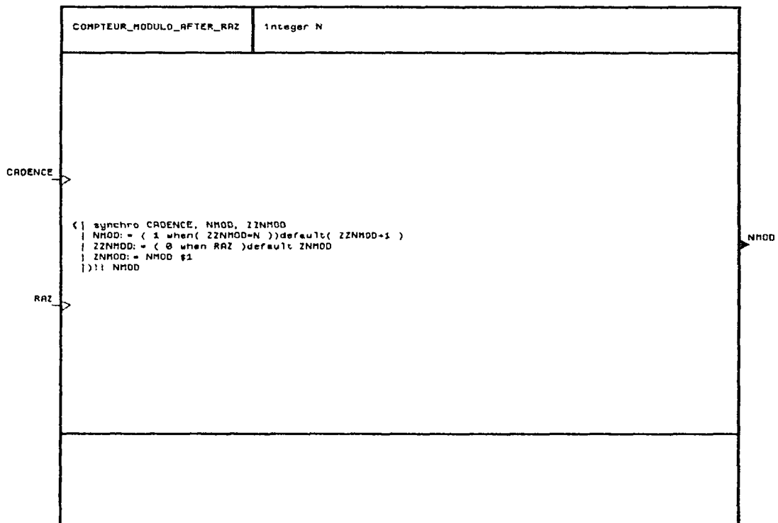
Figure B.7 : Le processus COMPTEUR_MODULO_AFTER_RAZ
