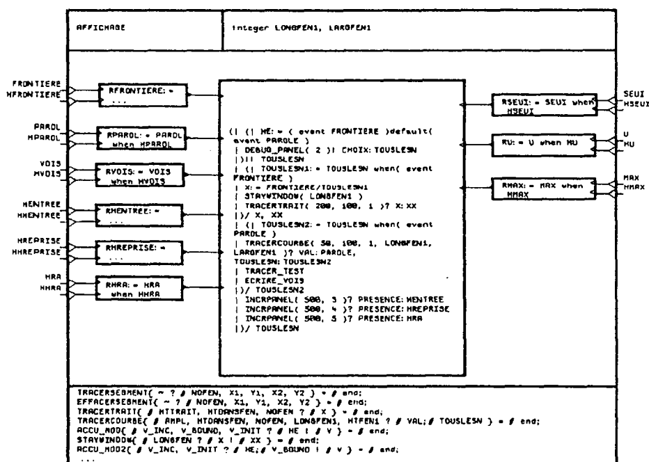
Figure V.2 : Le processus AFFICHAGE .
