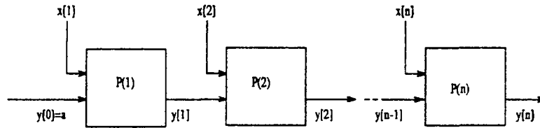
Figure III.7 : Block-diagramme d'un tableau régulier de processus
