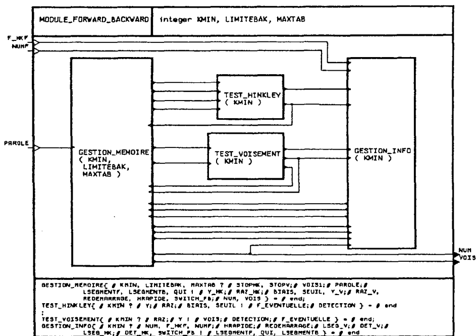
Figure IV.14 : Le processus MODULE_FORWARD_BACKWARD
