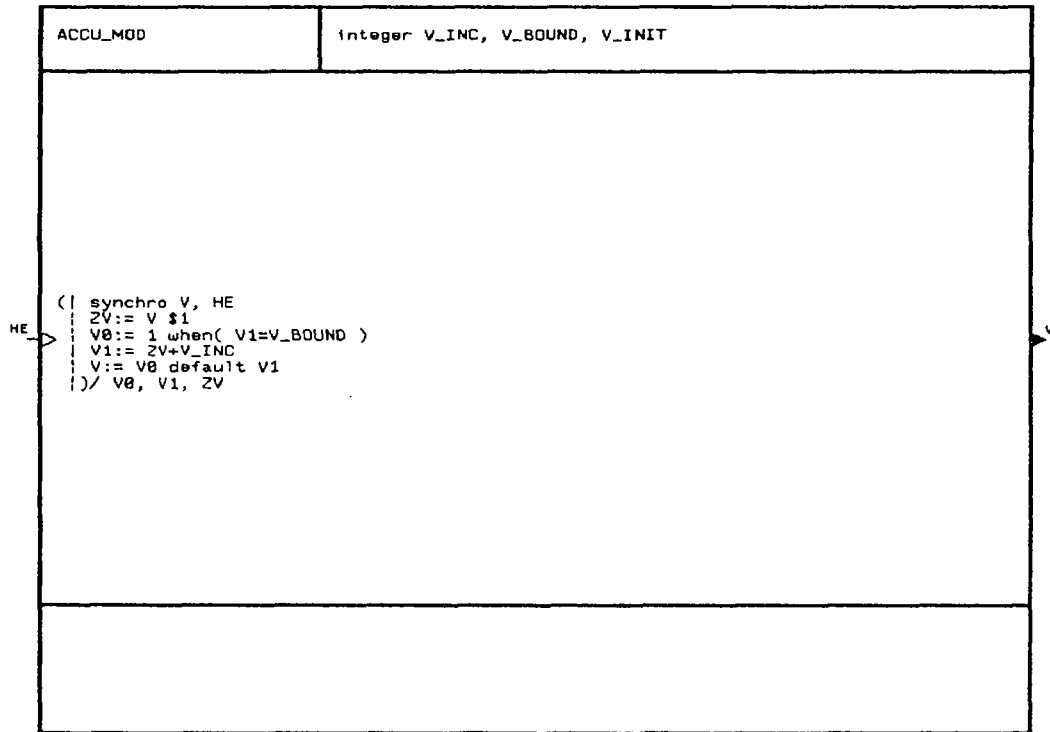
Figure B.5 : Le processus ACCU_MOD
