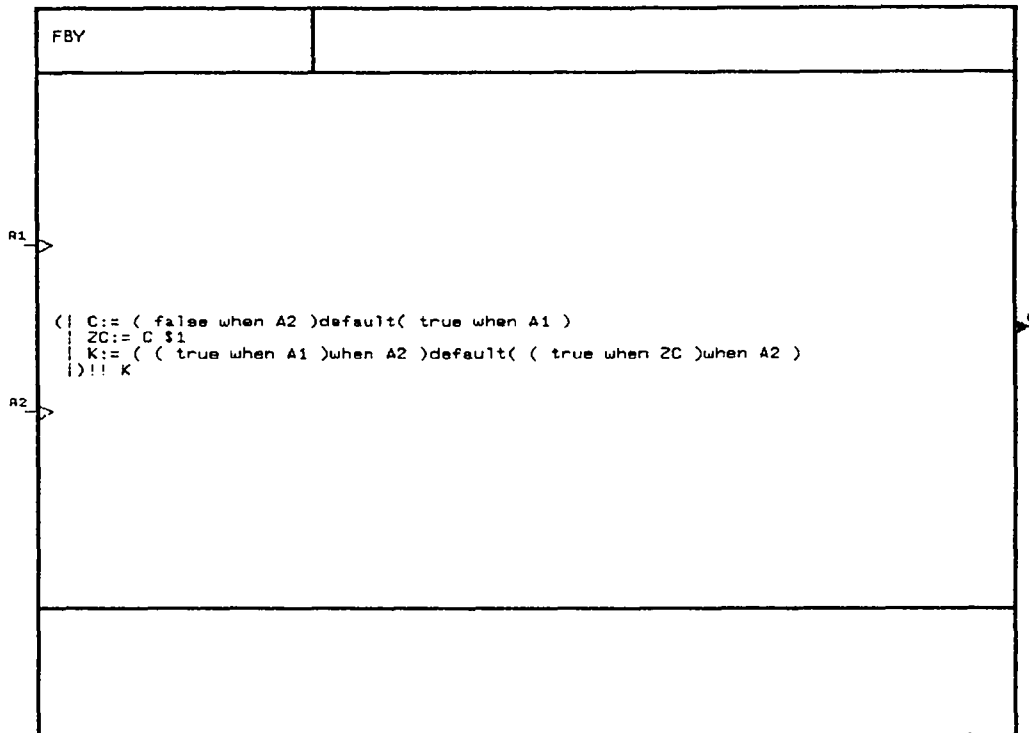
Figure B.10 : Le processus FBY
