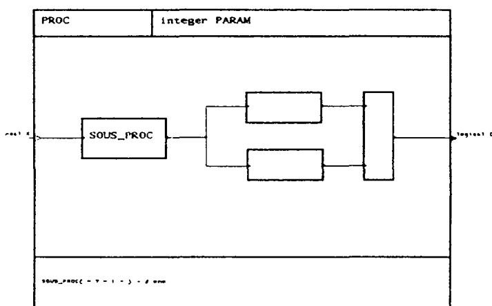
Figure III.1 : Vue graphique d'un processus de nom PROC. Les boîtes représentent les processus, les fils représentent les liens entre les signaux d'entrée/sortie. Dans cet exemple, X est un port d'entrée et C un port de sortie. Une zone est réservée pour le passage de paramètres (ou constantes): ici Param. De même une zone est réservée pour la déclaration des sous-processus: ici SOUS_PROC
