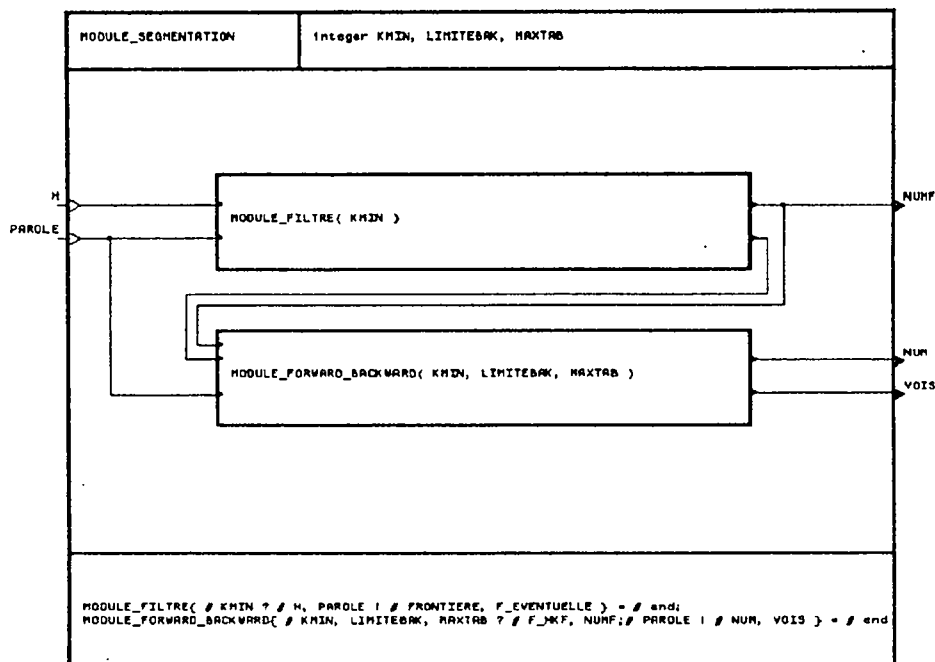
Figure IV.7 : Le module de segmentation
