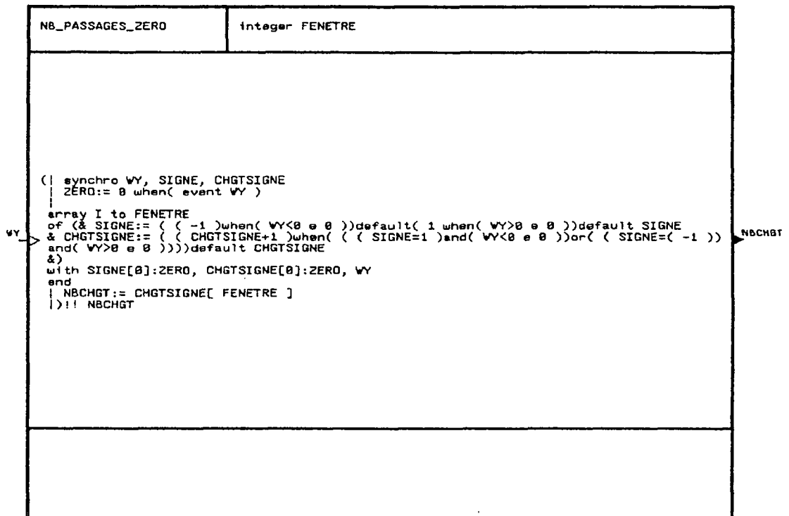
Figure A.1 : Le processus NB_PASSAGES_ZERO
