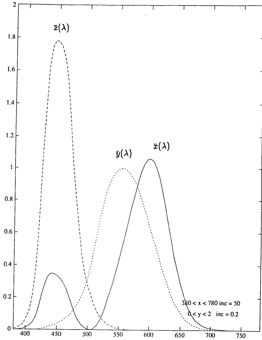
Figure 2.1 : Coefficients de distribution du système XYZ
