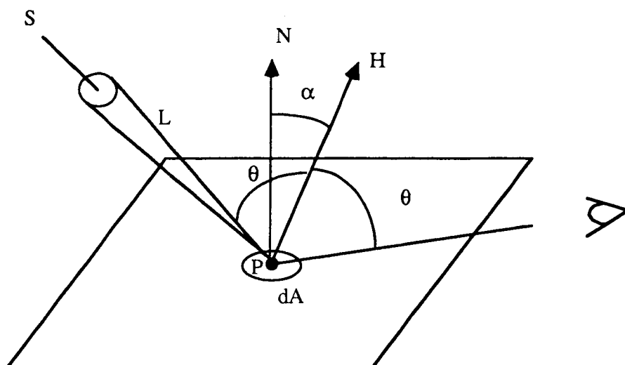
Figure 3.3 : Réflexion de la lumière sur une surface
