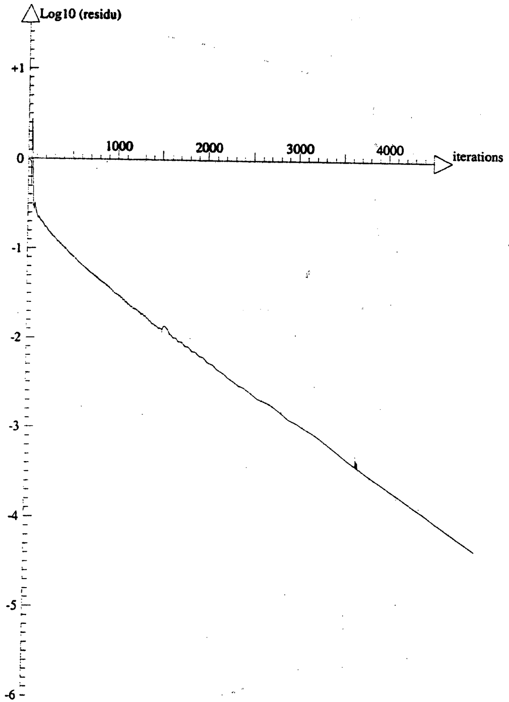
figure 8.h Ecoulement hypersonique d'un gaz réactif sur une sphère Convergence itérative , CFL = 0.4
