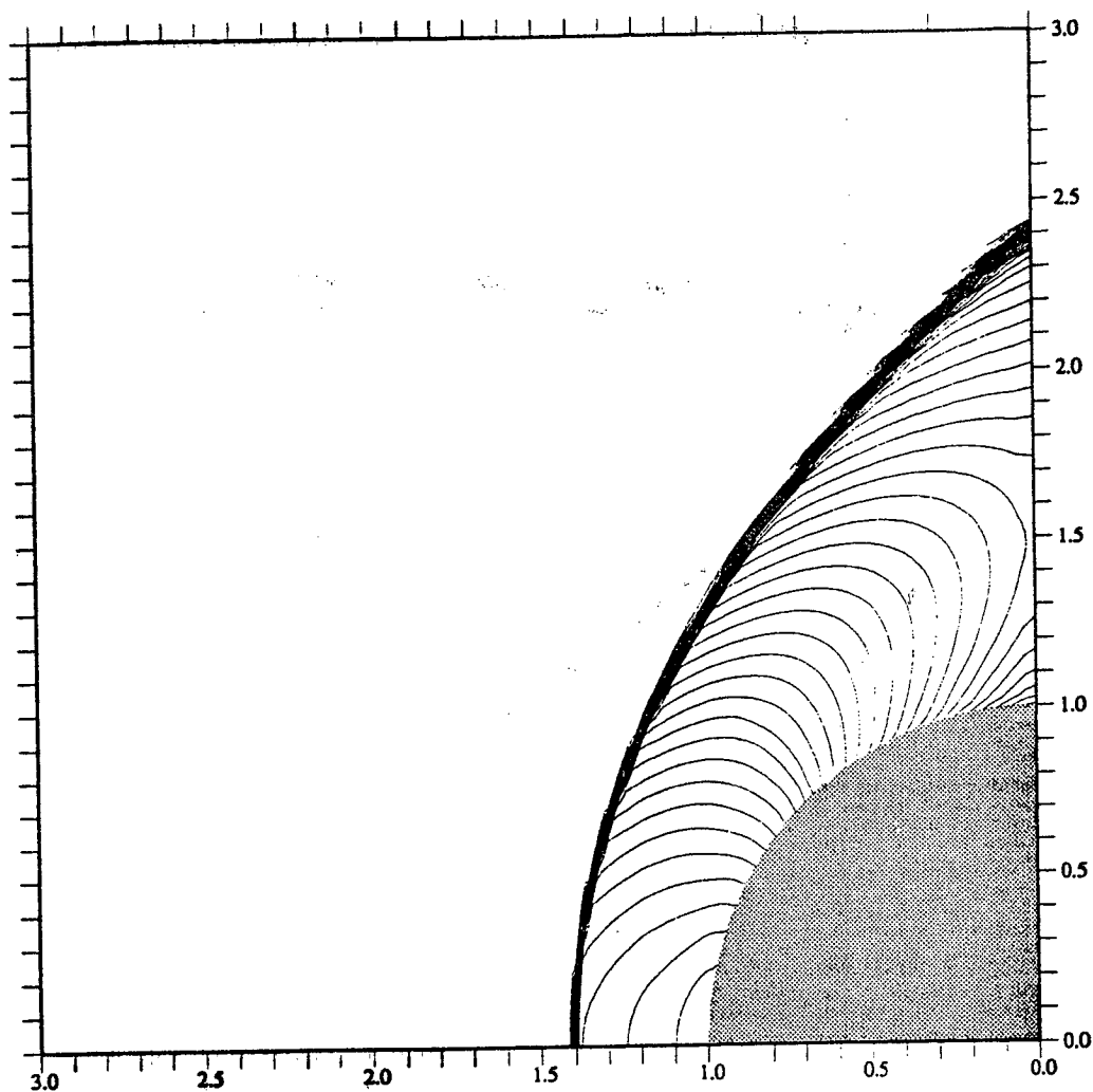
figure 4.d Écoulement hypersonique d'un fluide parfait sur un cylindre lignes iso-température ( M_\infty = 25 )
