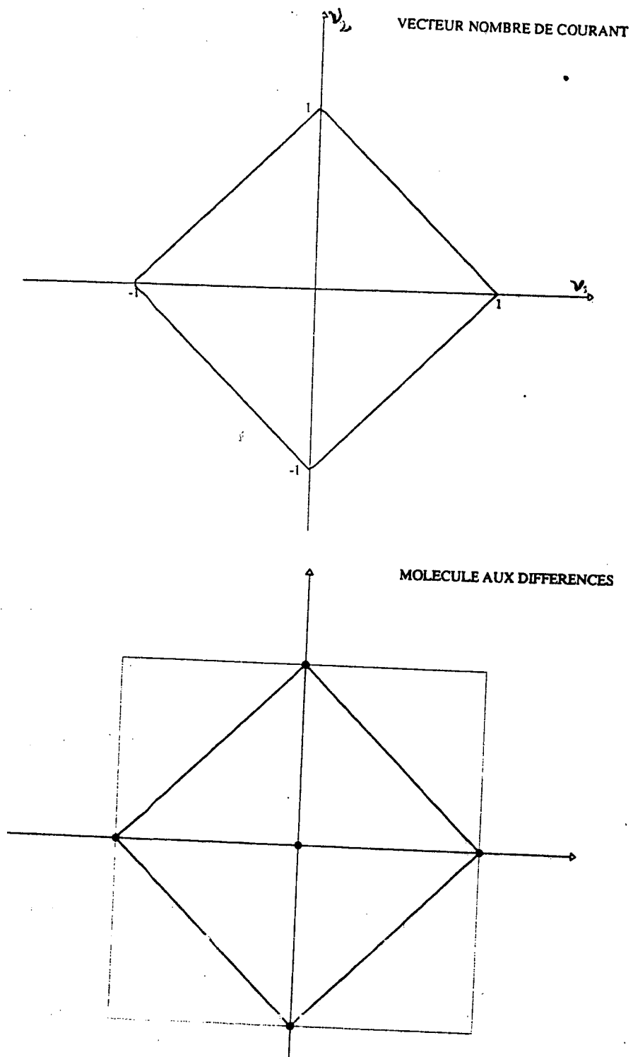
Figure 2 Domaine de stabilité d'un schéma d'ordre 1
