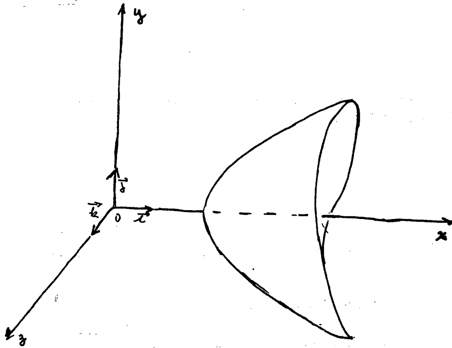
Figure 1.1 Domaine axisymétrique \Omega et perturbé \Omega_\epsilon associé
