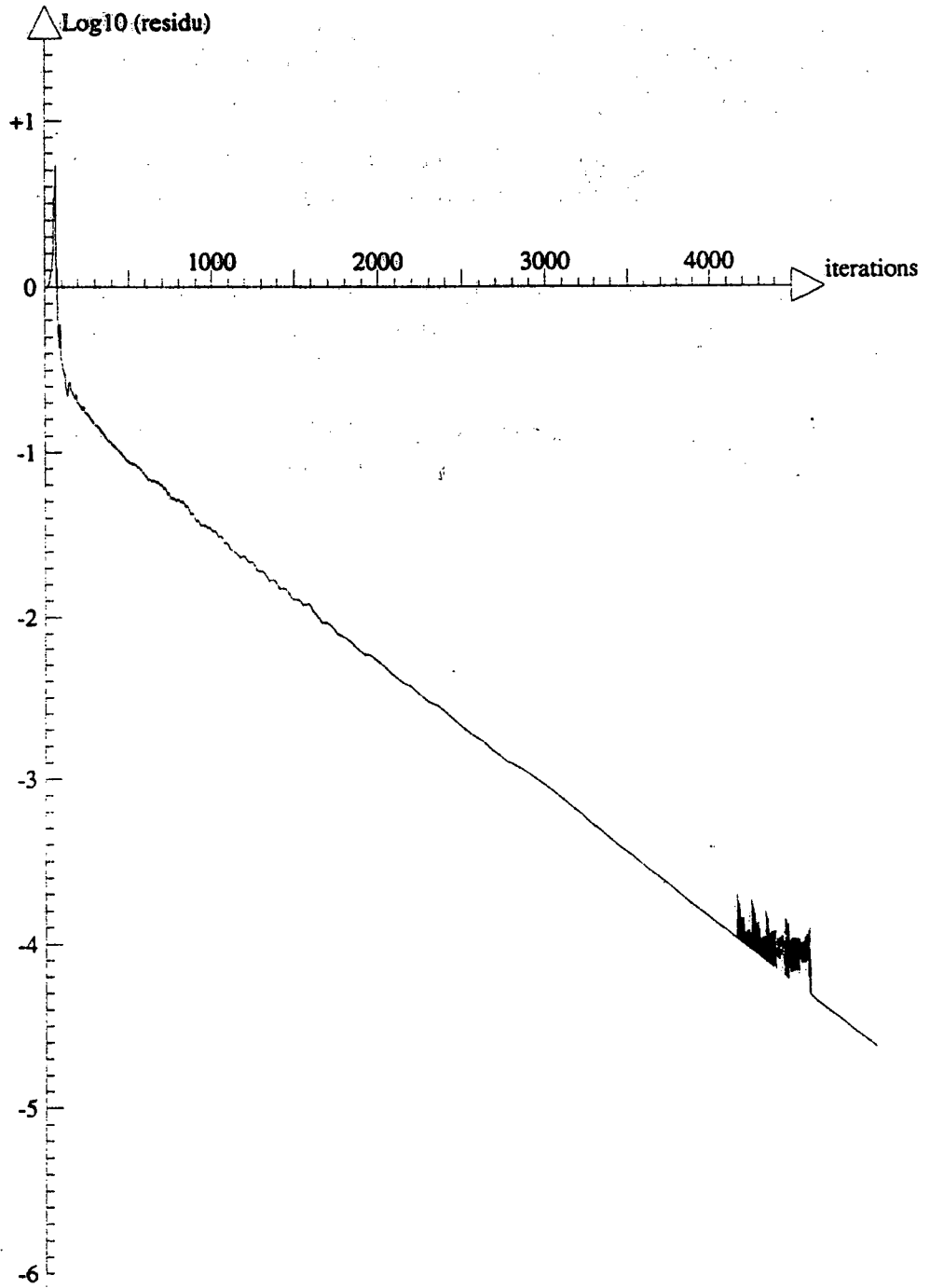
figure 10.g Ecoulement hypersonique d'un gaz réactif sur une sphère Convergence itérative , CFL = 0.4
