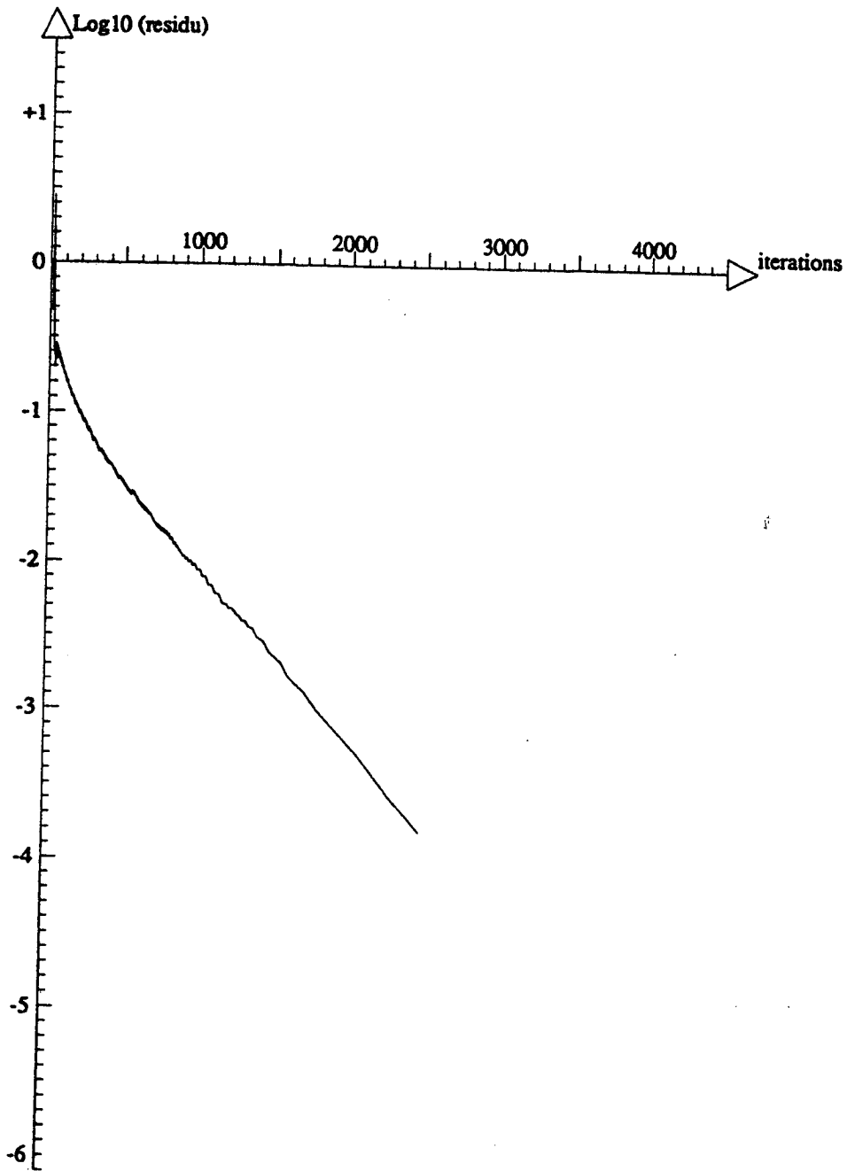
figure 3.d Ecoulement hypersonique d'un fluide parfait sur un cylindre Convergence itérative ( CFL = 0.4 )
