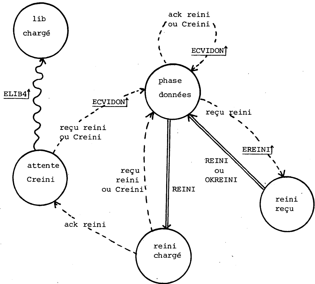
Figure IV.19. - AUTOMATE SIGNALISATION : REINITIALISATION.
