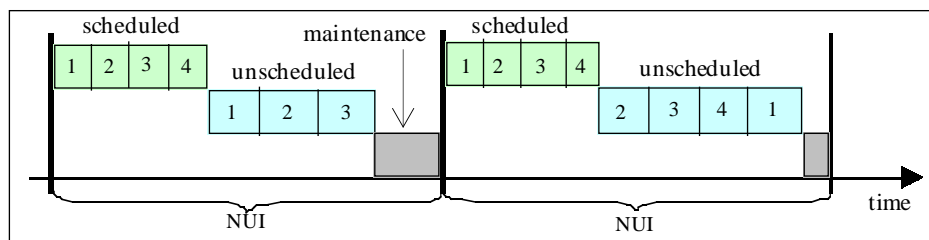
Fig. 1. ControlNet protocol.
