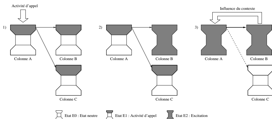
Figure 4. 1) La colonne A reçoit une activité d'appel externe (une colonne voisine par exemple) qui est transmise aux colonnes voisines (ici, les colonnes B et C). 2) Le contexte actuel autorise l'excitation de la colonne B (par exemple, un mouvement moteur peut être déclenché). 3) Le changement de contexte induit par l'activation de la colonne B autorise l'excitation de la colonne A. Le lien d'appel de la colonne A vers la colonne B est renforcé alors que celui vers la colonne C est diminué. La colonne A "apprend" ainsi qu'il est préférable d'appeler la colonne B pour pouvoir être excitée
