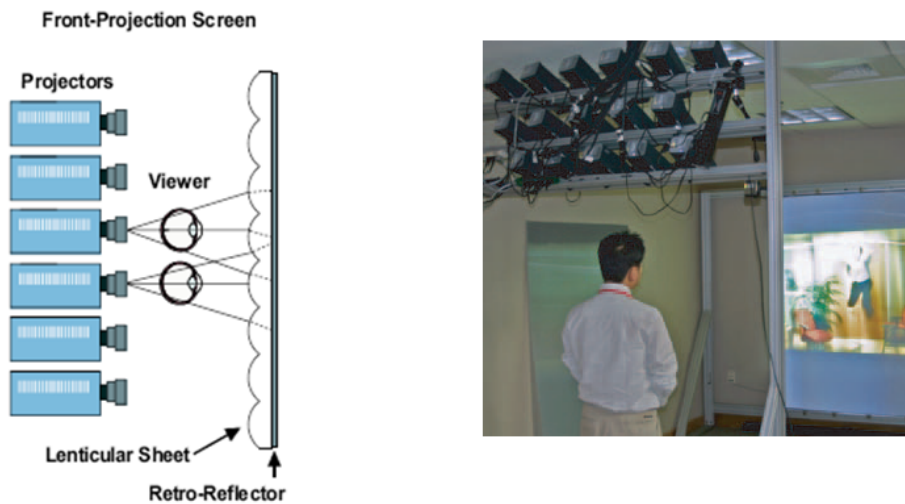
FIG. 10 – Système de retransmission TV 3D composé de 16 vidéo-projecteurs et d'un écran de projection miroir équipé d'un simple panneau lenticulaire.
