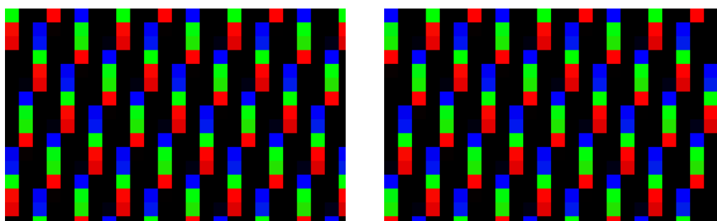
FIG. 32 – Utilisation du vrai motif d'entrelacement. A gauche, image entrelacée représentant la vue 1 blanche et les autres vues noires. A droite, image entrelacée représentant la vue 2 blanche et les autres vues noires.
