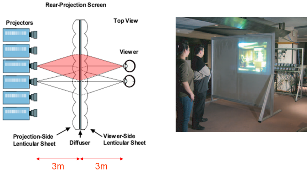
FIG. 9 – Système de retransmission TV 3D composé de 16 vidéo-projecteurs et d'un écran de projection diffuseur équipé d'un double panneau lenticulaire (de chaque côté de l'écran).
