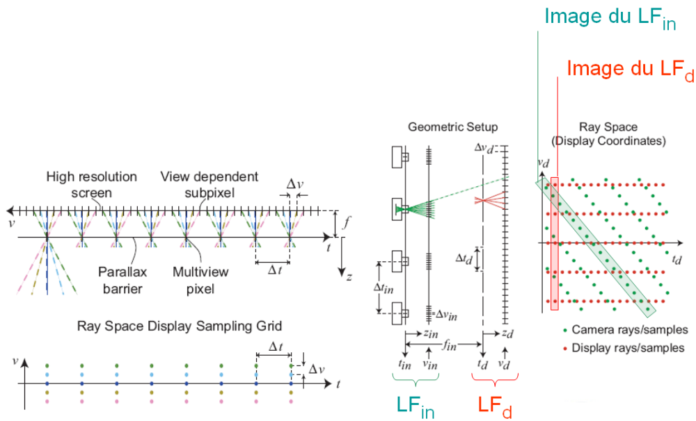
FIG. 22 – À gauche, analogie entre un écran 3D à barrière de parallaxe et un lumigraphe; À droite : reprojection d'un lumigraphe pré-acquis LF_{in} pour construire le lumigraphe réellement affiché LF_d .
