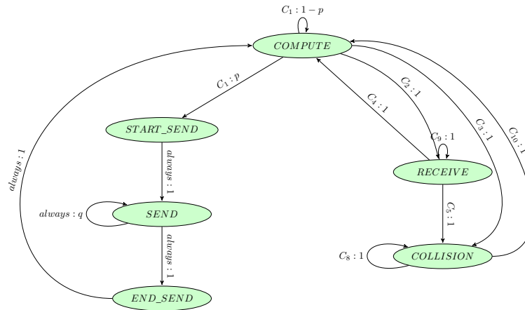
Figure 1. Exemple d'automate
