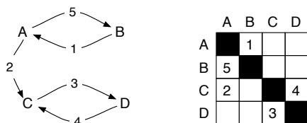
Figure 10: Une matrice de dépendance correspondant au graphe à gauche.
