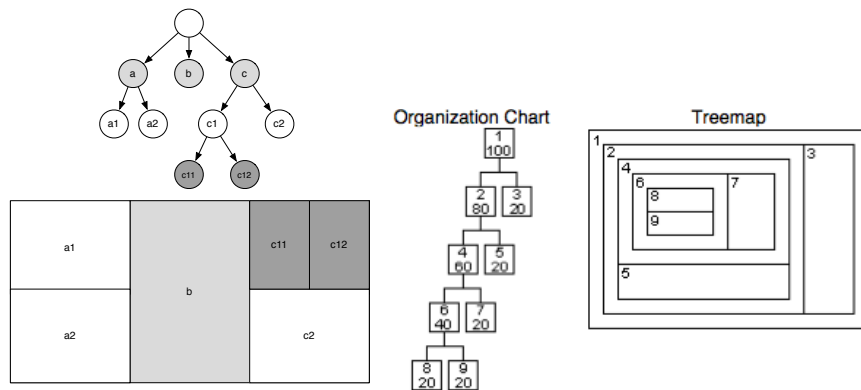
Figure 2: (gauche) Une TreeMap montrant 6 nœuds répartis sur 4 niveaux hiérarchiques (droite) Comparer une TreeMap et un arbre organisationnel (pris dans l'article [BN01]).
