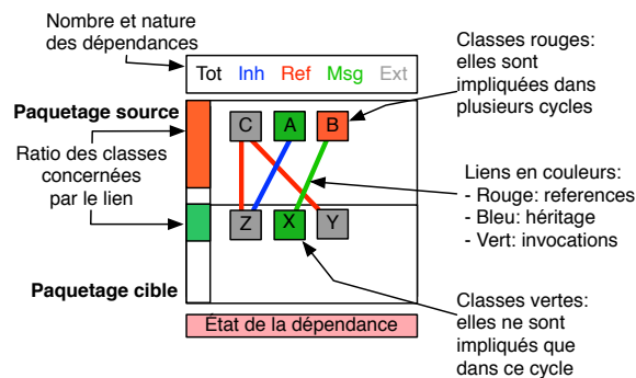
Figure 12: Cellule représentant un lien entre deux paquetages.
