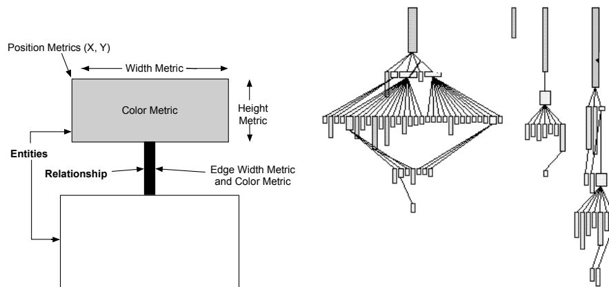
Figure 4: (Gauche) Principe de Polymetric Views. (Droite) System complexity. Largeur: NOA. Hauteur: NOM. Couleur: WLOC.
