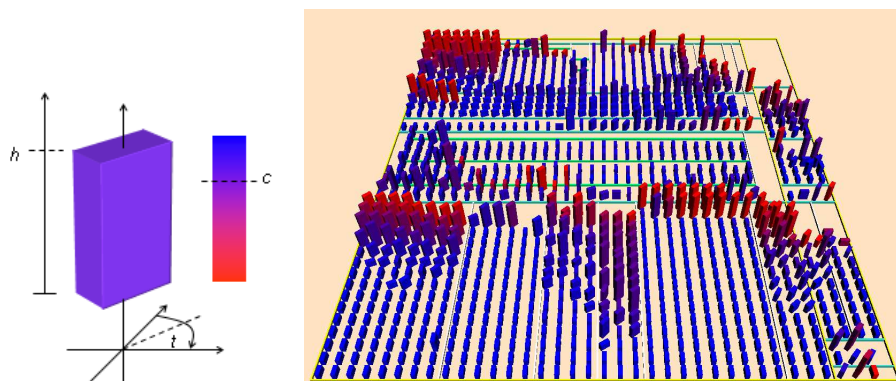
Figure 3: (Gauche) boîte 3D représentant un élément dans Verso, il y a 3 dimensions (hauteur, angle, couleur). (Droite) Visualisation de classes organisées par paquetage.
