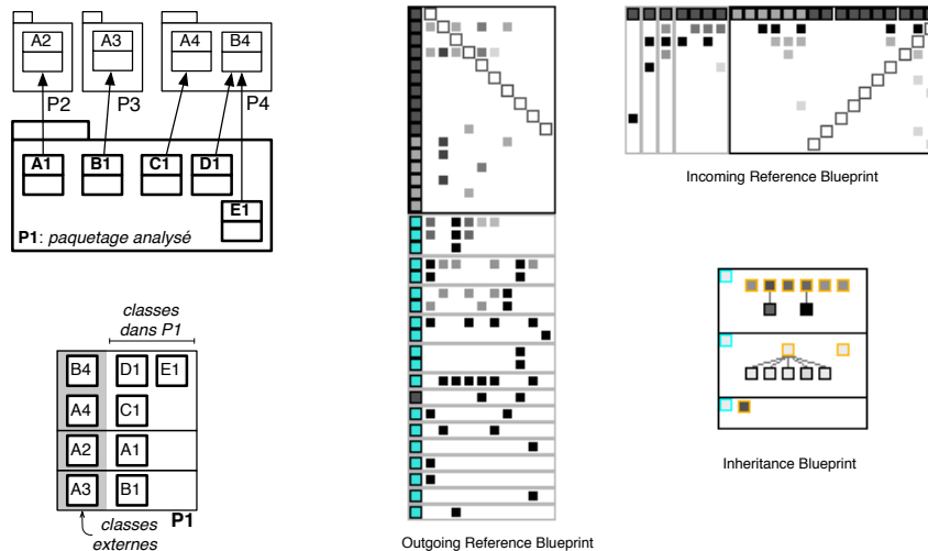
Figure 9: (Gauche) Principe de Package Blueprint avec 4 paquetages. (Droite) Les trois visualisations de Package Blueprint en œuvre.
