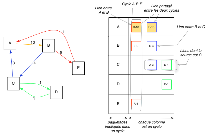
Figure 16: (Gauche) un graphe cyclique. (Droite) Structure de sa CycleTable.
