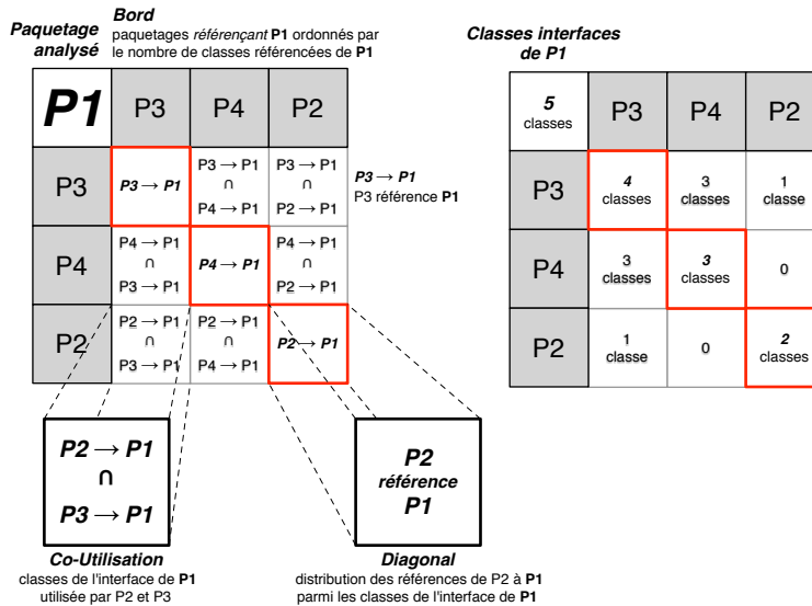
Figure 5: Structure d'un fingerprint entrant pour le package P_1 .
