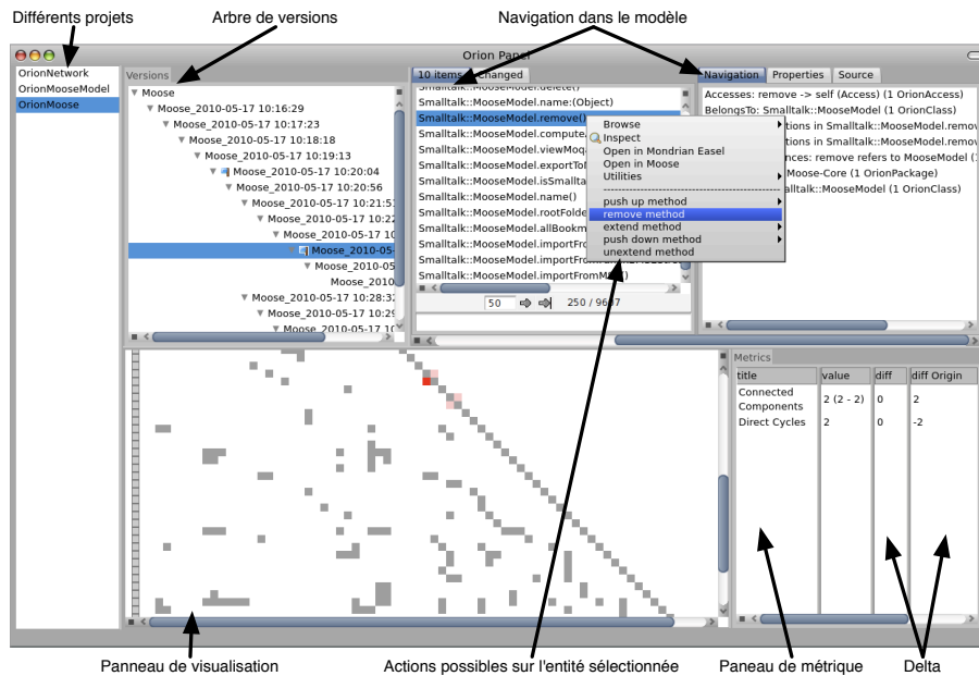
Figure 20: Un navigateur Orion, dédié à la suppression des cycles entre paquetages.
