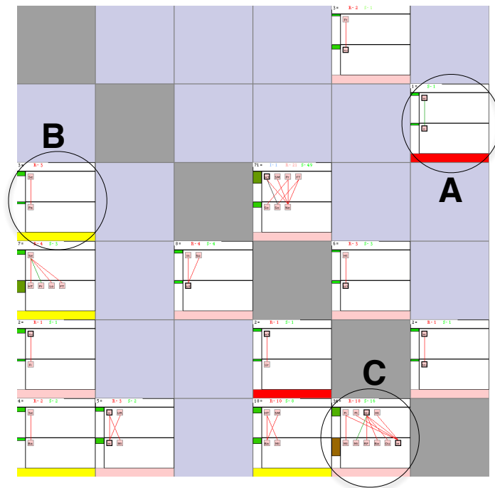
Figure 15: Aperçu d'une eDSM: A– dépendance à supprimer, B– dépendance faisant partie d'un cycle non direct, C– cette dépendance a de nombreuses relations.
