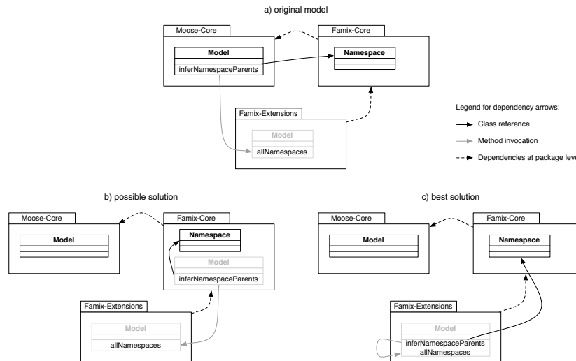
Figure 18: a) deux cycles entre trois paquetages; b) un changement qui enlève les deux cycles mais en crée un nouveau; c) un changement qui enlève les deux cycles.
