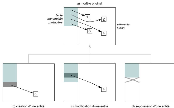
Figure 19: Le système de partage d’Orion : illustration des différents changements (création, modification, suppression)
