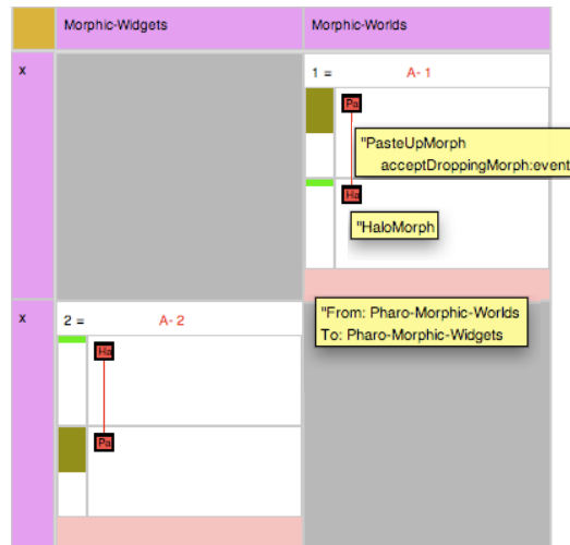
Figure 13: Deux cellules représentant un cycle direct, les infobulles informent des méthodes concernées par le lien.
