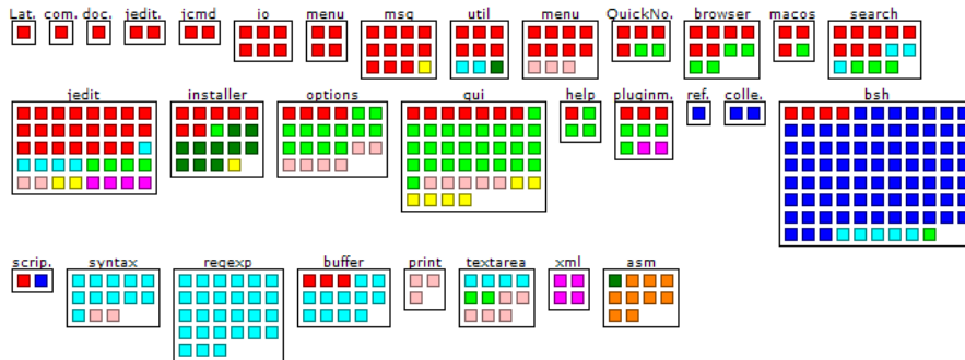
Figure 8: DistributionMap de JEdit montrant les "Core Classes" (rouge), les "UI Classes" (vert), les "Scripting classes" (bleu)
