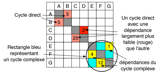
Figure 14: Une DSM colorée.
