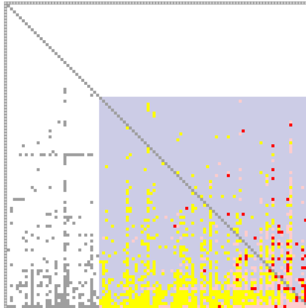
Figure 11: La DSM de Pharo1.0: le carré bleu représente un ensemble de paquetages en cycle, en rouges les cycles directs, en jaune et en gris les dépendances simples.
