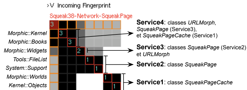
Figure 6: Incoming Fingerprint du paquetage SqueakPage package du sous-système Squeak38::Network .
