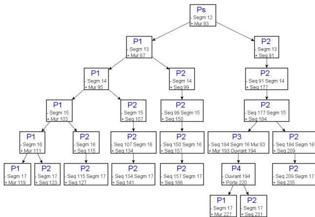
(a) Phase de construction de l'arbre d'analyse de l'étape n (segment 12), déduite de la Figure 5(a)
