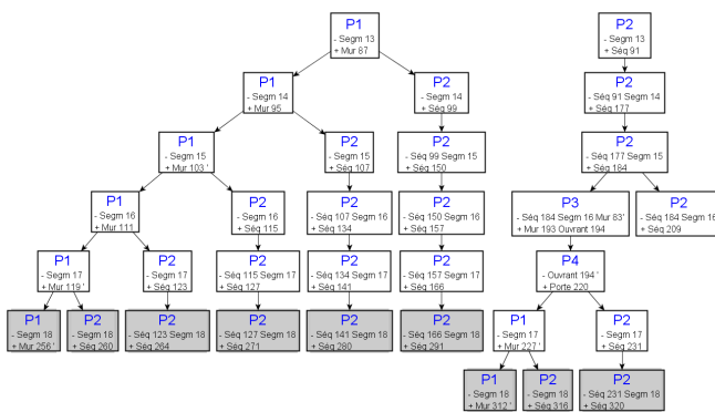
(b) Phase de construction de l'arbre d'analyse de l'étape n+1 (segment 13), déduite de la Figure 5(b). Les nœuds grisés indiquent les nouvelles règles de production appliquées en déplacement le contexte local.
