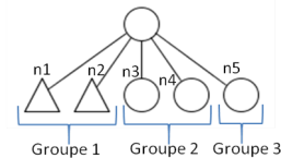
(b) Méthode de construction de l'arbre d'analyse de IMISketch optimisé . Le nombre de nœuds nouvellement créés = 6. Les fils directs de la racine sont groupés par éléments consommés.
