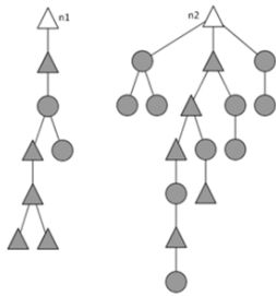
(b) Méthode de construction de l'arbre d'analyse de IMISketch optimisé . Les racines n1 et n2 développées appartiennent au même groupe (Groupe 1) (elles partagent les mêmes éléments consommés). Le nombre de nœuds nouvellement créés = 22
