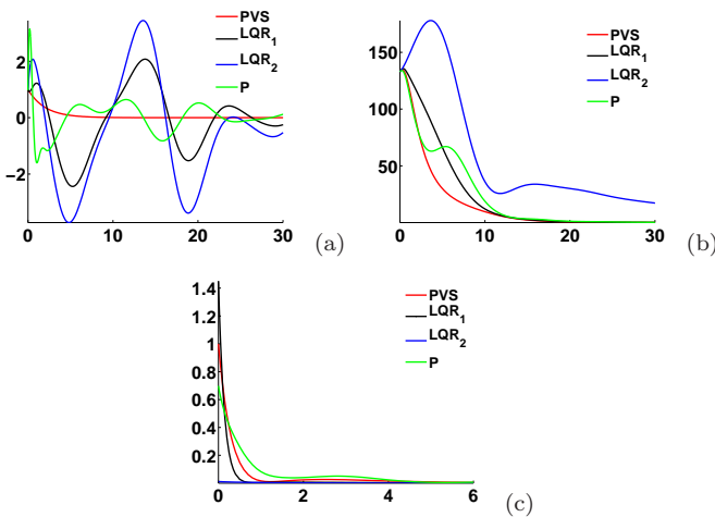
FIG. 6. (a) Trainée en fonction du temps; (b) densité d'énergie cinétique en fonction du temps (c) Norme du signal de commande u(t) en fonction du temps (axe des abscisses en seconde).
