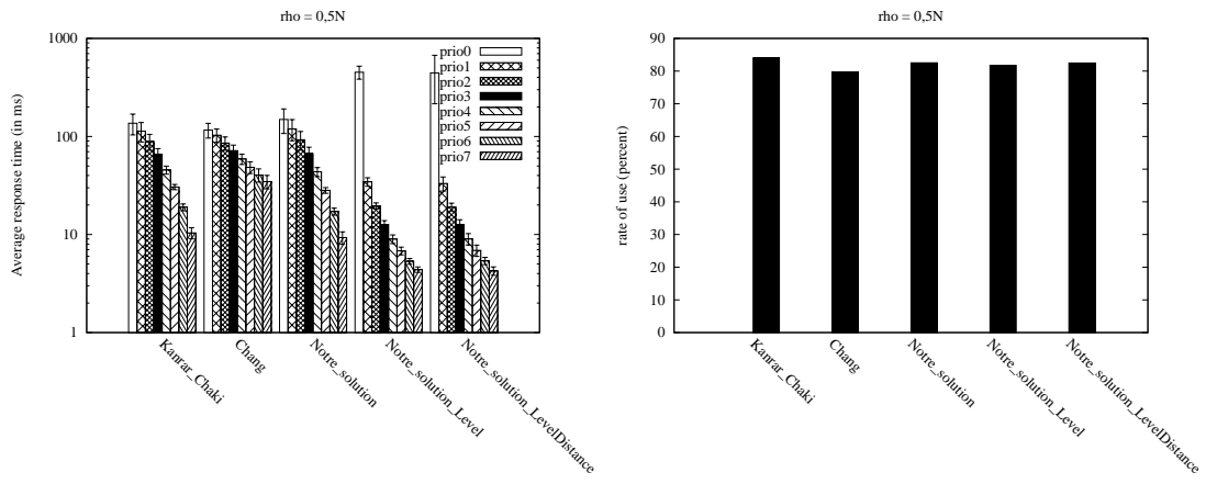
(c) Temps de réponse moyen pour entrer en section critique par priorité (d) Taux d'utilisation de la section critique
