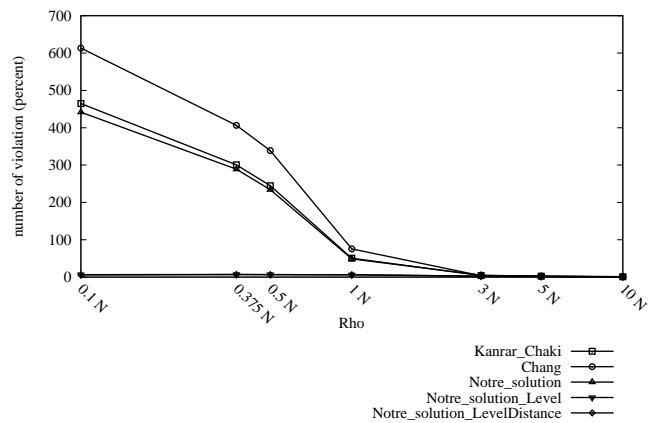
(c) Nombre total de violations en pourcentage de requêtes
