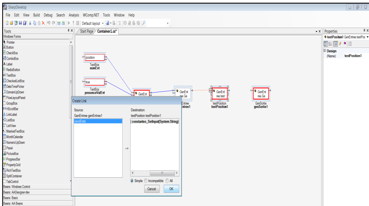
Figure 38: liaison générateur d'entrée/moniteur synchrone
