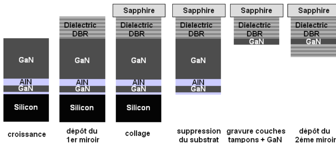
FIG. 4.1 – Étapes de fabrication de la microcavité complètement hybride (échantillon A611).
