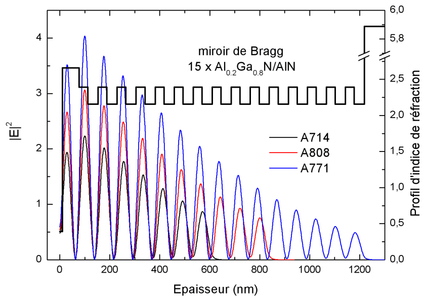
FIG. 3.4 – Profil d'indice et carré du module du champ électrique pour les échantillons A714, A808 et A771.
