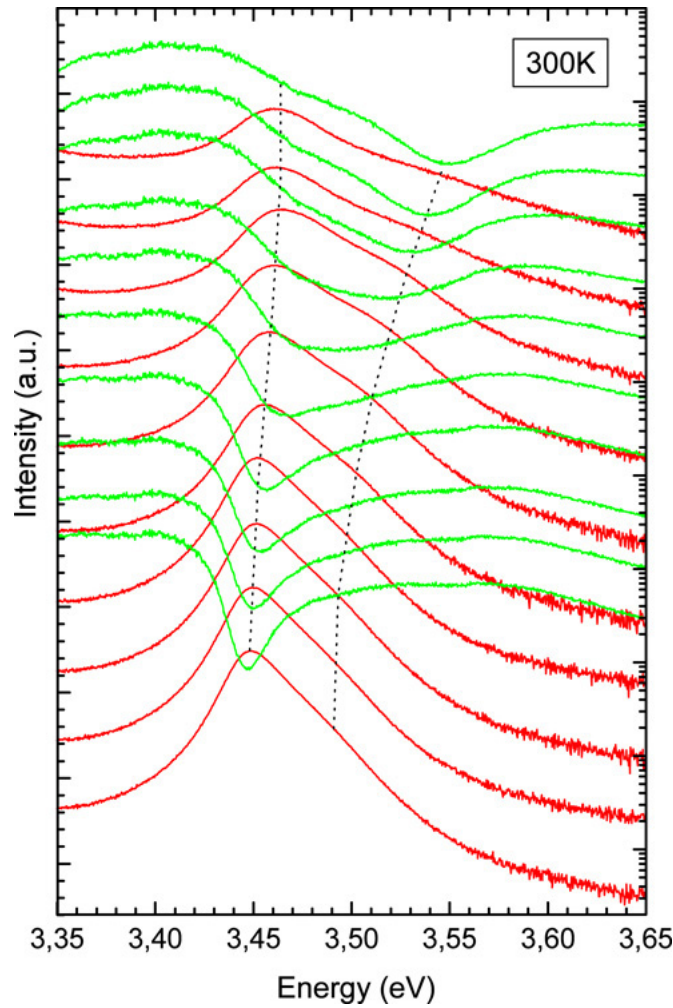
FIG. 3.17 – Réflectivité et photoluminescence en position sur l'échantillon A808D à 300K [73].
