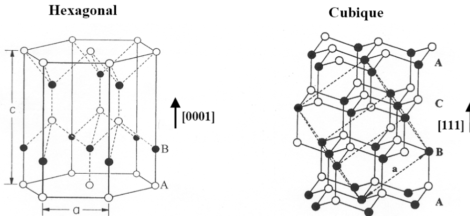
FIG. 1.2 – Arrangement des atomes de Ga (cercle vide) et N (cercle plein) de la maille cristalline des structures hexagonale et cubique [14].
