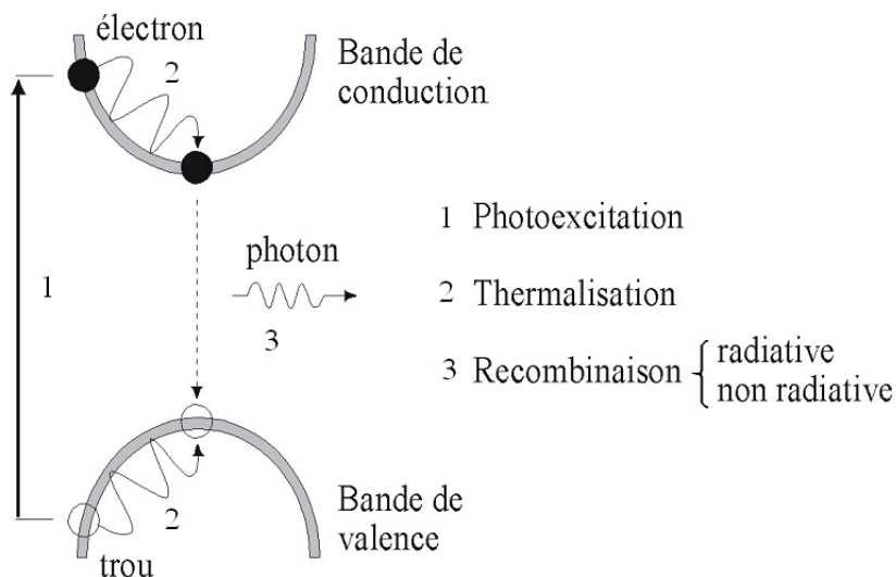
FIG. 2.4 – Processus mis en jeu en photoluminescence d'après la référence [58].
