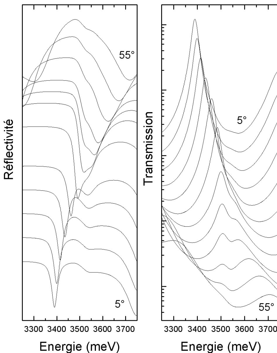
FIG. 4.15 – Simulation de réflectivité et transmission en angle de 5^\circ à 55^\circ par pas de 5^\circ (excepté pour la résonance \theta=37.5^\circ ) pour la polarisation TM à 5 K.
