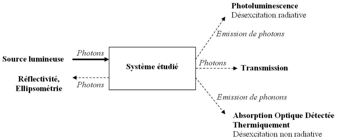
FIG. 2.1 – Techniques de spectroscopie optique.
