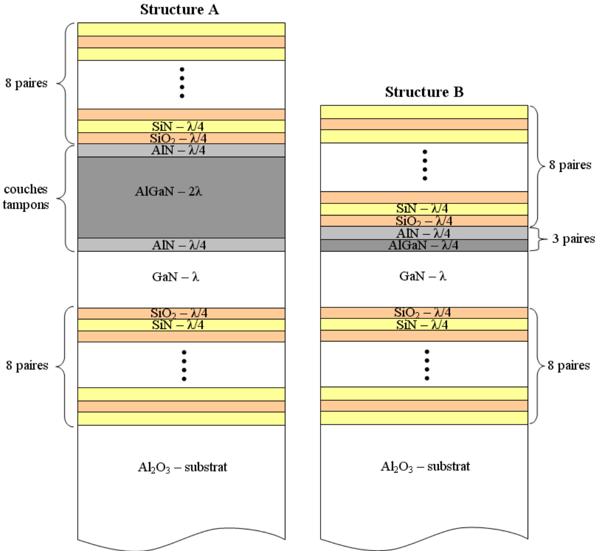
FIG. 4.19 – Schéma des structures A et B.
