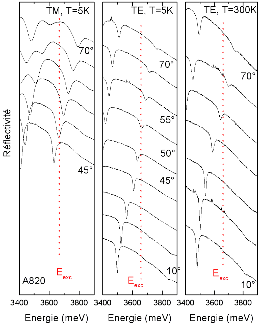
FIG. 3.32 – Spectres de réflectivité en angle pour la cavité complète A820 à 5 K et 300 K.
