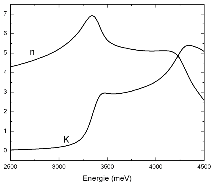
FIG. 2.17 – Parties réelle et imaginaire de l'indice complexe de silicium en fonction de l'énergie.
