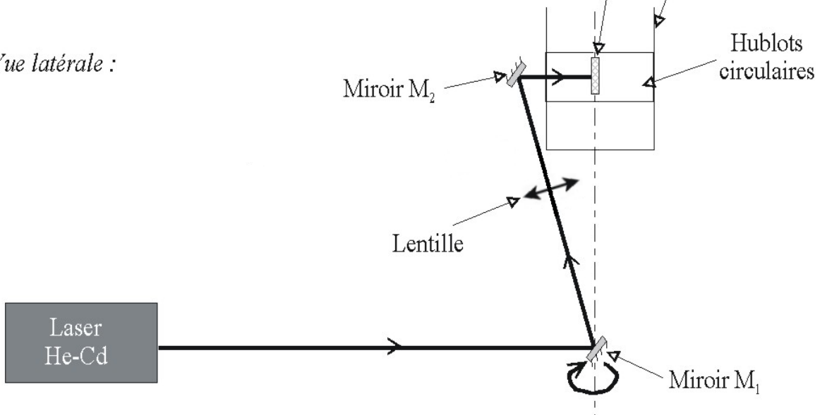
FIG. 2.5 – Schéma du spectromètre de photoluminescence résolue en angle [58].
