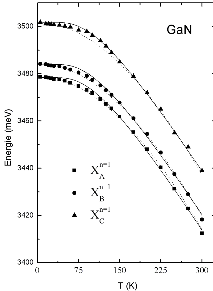
FIG. 1.7 – Évolution des énergies des excitons A, B et C en fonction de la température d'après la référence [29].
