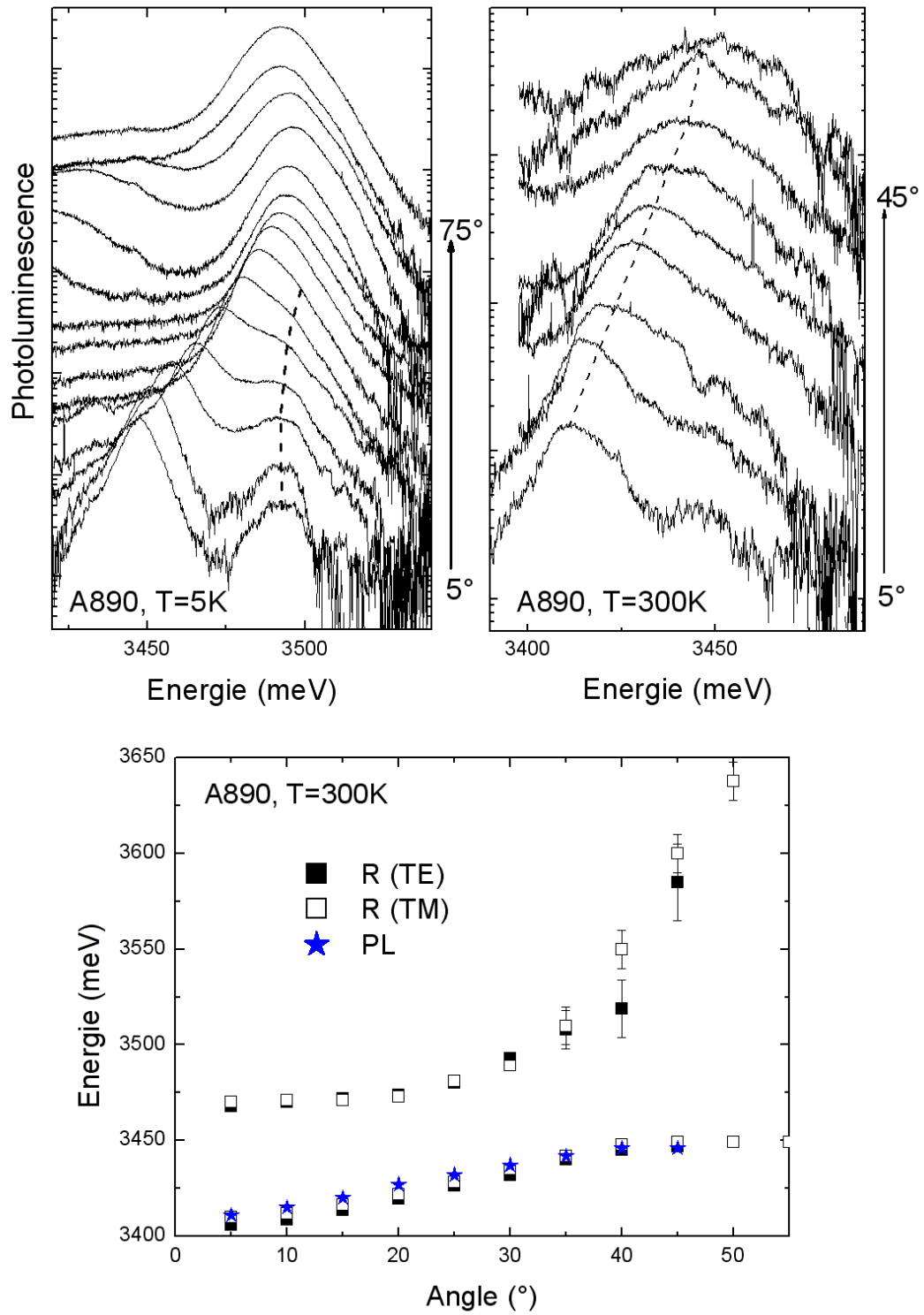
FIG. 3.26 – Spectres de photoluminescence résolue en angle à T=5 K et 300 K ainsi que la dispersion des modes polaritoniques à 300 K.
