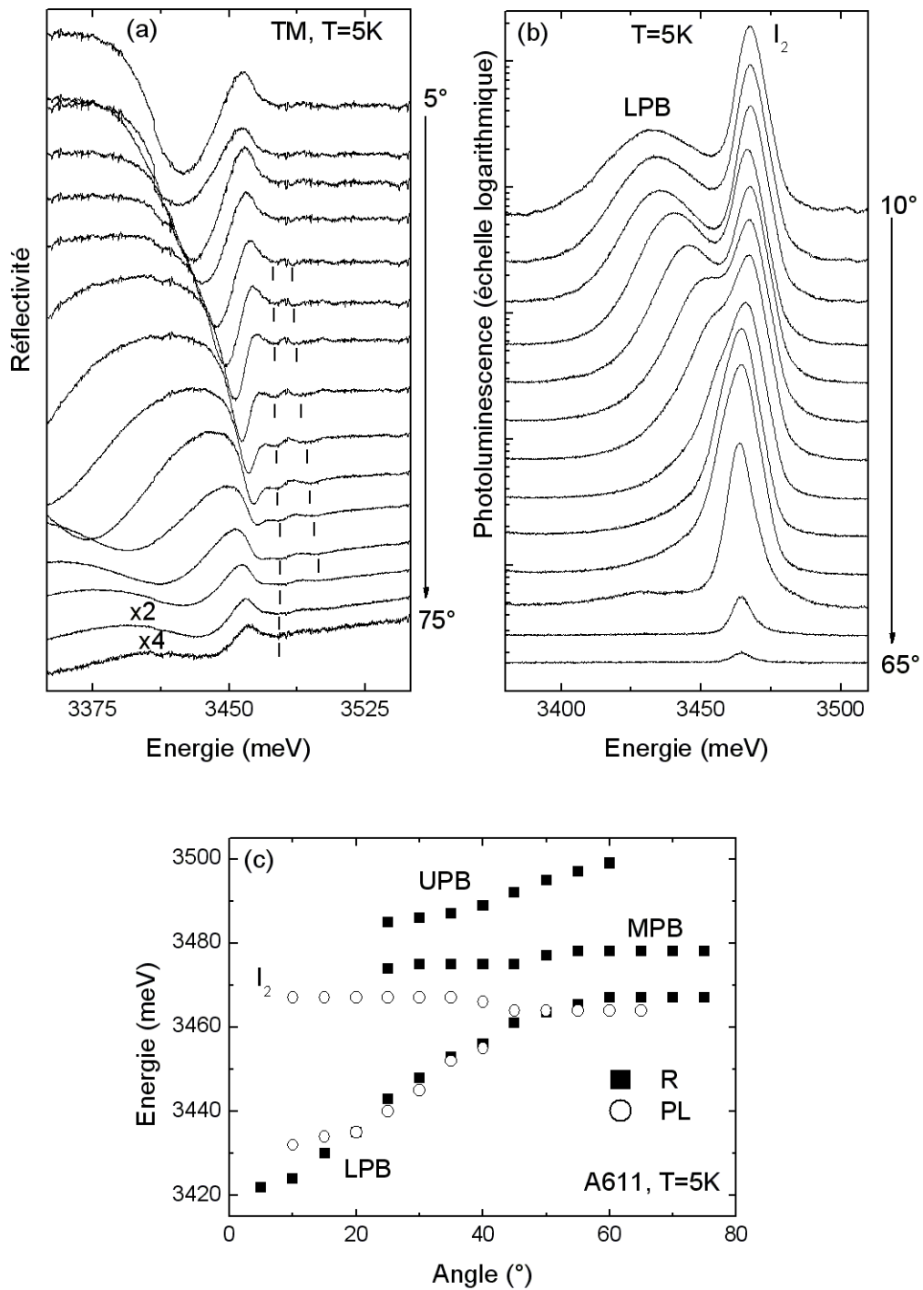
FIG. 4.2 – (a) Spectres de réflectivité en angle en polarisation TM à T=5 K de 5^\circ à 75^\circ par pas de 5^\circ . (b) Spectres de photoluminescence en angle à T=5 K de 10^\circ à 65^\circ par pas de 5^\circ . (c) Courbes de dispersion.
