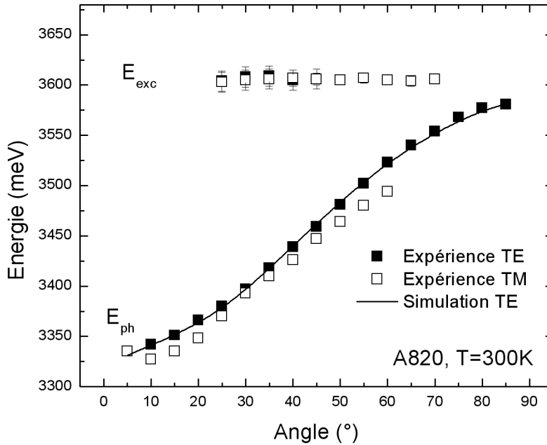
FIG. 3.31 – Évolution des modes excitonique et photonique en fonction de l'angle d'incidence pour la demi-cavité A820 à 300K pour les deux polarisations et simulation avec les matrices de transfert de la dispersion photonique en polarisation TE.
