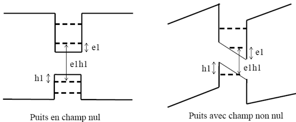
FIG. 3.34 – Influence d'un champ électrique sur les états électroniques d'un puits quantique (effet Stark) [14].
