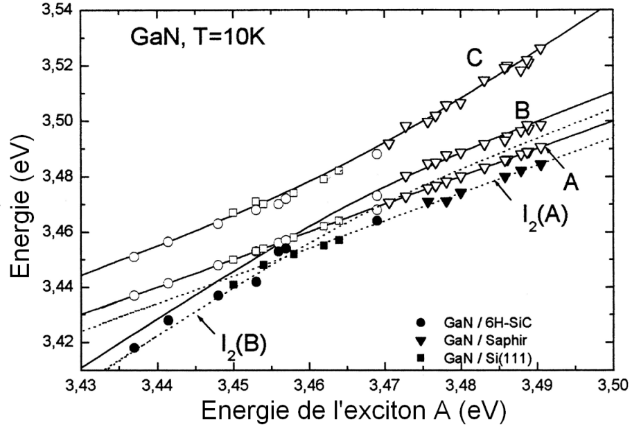
FIG. 1.6 – Énergie des excitons libres A, B, C et des excitons liés I_2 en fonction de l'énergie de l'exciton A pour différents échantillons de GaN épitaxiés sur substrat saphir, 6H-SiC et Si d'après la référence [24].
