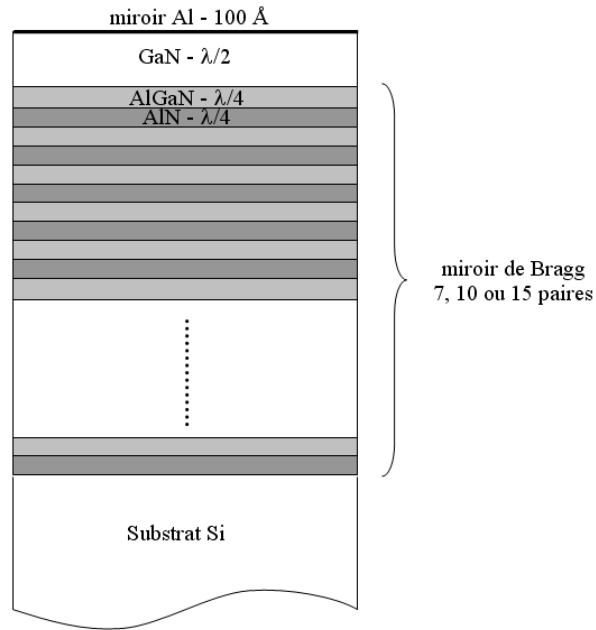
FIG. 3.3 – Schéma des structures A714 (7 paires), A808 (10 paires) et A771 (15 paires).
