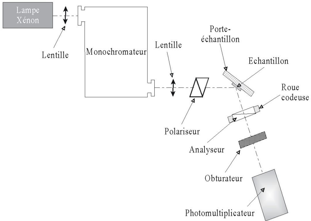
FIG. 2.6 – Schéma du spectromètre d'ellipsométrie.
