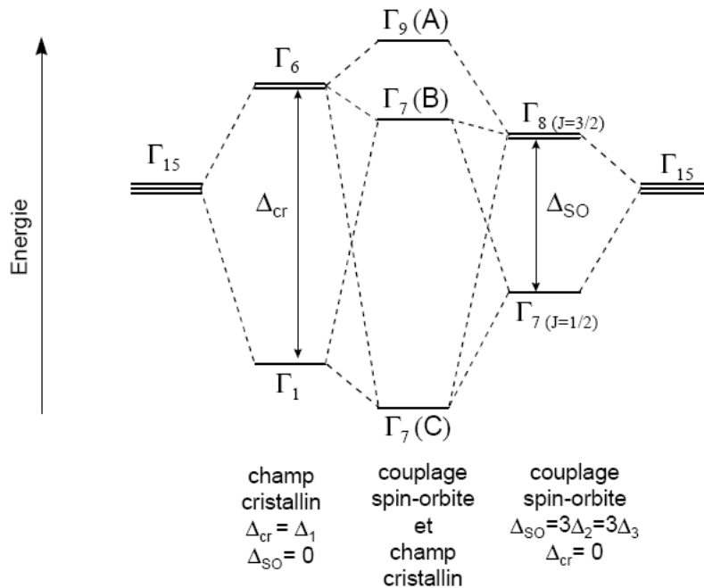
FIG. 1.4 – Représentation des bandes de valence de GaN hexagonal au point \Gamma ( k=0 ) [23].
