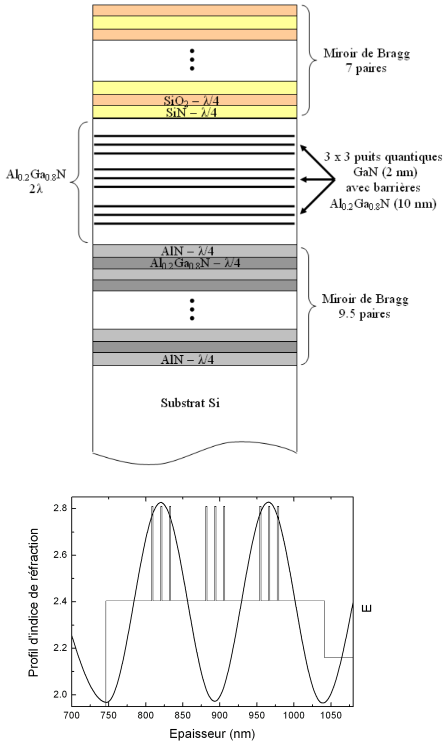
FIG. 3.28 – Schéma de la structure A820 et répartition des puits par rapport au champ électrique dans la cavité.
