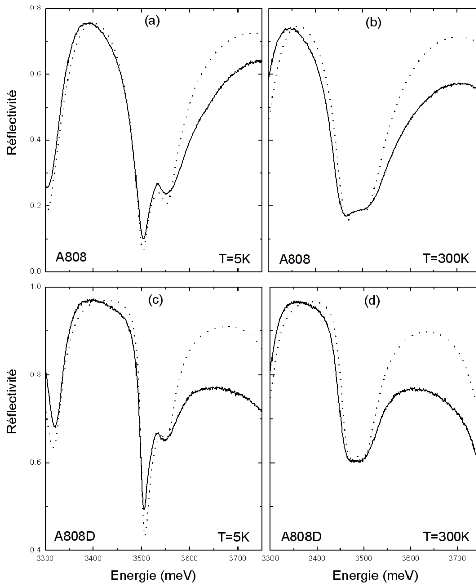
FIG. 3.38 – Simulations avec les matrices de transfert (traits pointillés) et spectres expérimentaux de réflectivité (traits pleins) à 5 K et à 300 K pour les échantillons A808 (a-b) et A808D (c-d) en configuration de couplage fort.
