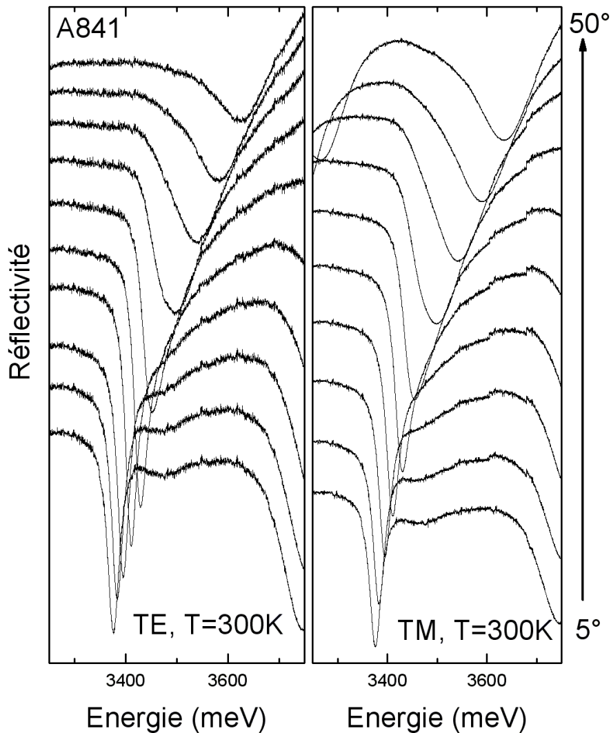
FIG. 4.12 – Spectres de réflectivité résolue en angle de 5^\circ à 50^\circ par pas de 5^\circ pour les polarisations TE et TM à température ambiante.
