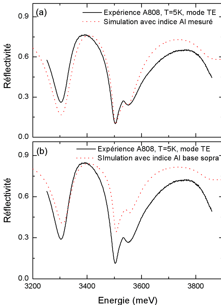
FIG. 2.16 – Ajustement d'un spectre de réflectivité (a) avec l'indice Al mesuré par ellipsométrie et (b) avec l'indice Al de la base Sopra.
