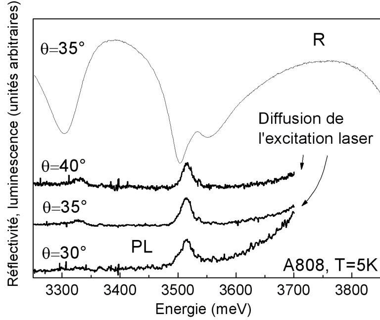
FIG. 3.8 – Spectres de réflectivité (R) à la résonance ( \theta=35^\circ ) et de photoluminescence (PL) pour \theta=30, 35 et 40^\circ à 5 K.
