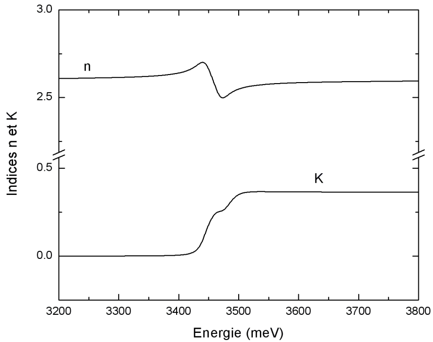
FIG. 2.13 – Calcul de l'évolution des parties réelle et imaginaire de l'indice de GaN.
