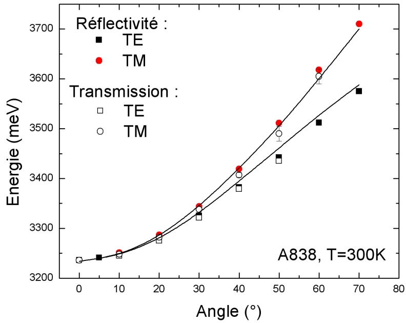
FIG. 4.10 – Dispersion du mode photonique mesurée en réflectivité et en transmission pour les polarisations TE et TM à T=300 K.
