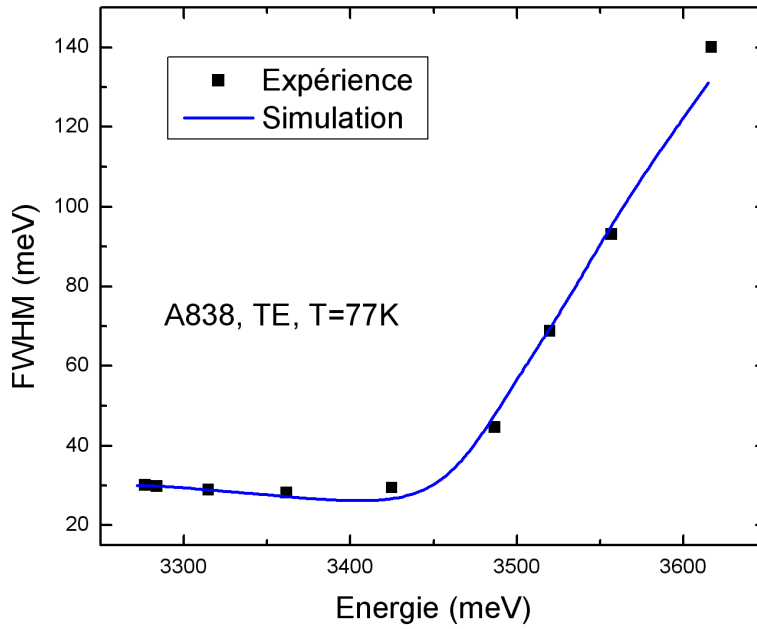
FIG. 4.11 – Largeur à mi-hauteur du mode optique en fonction de l'énergie en polarisation TE pour T=77 K.
