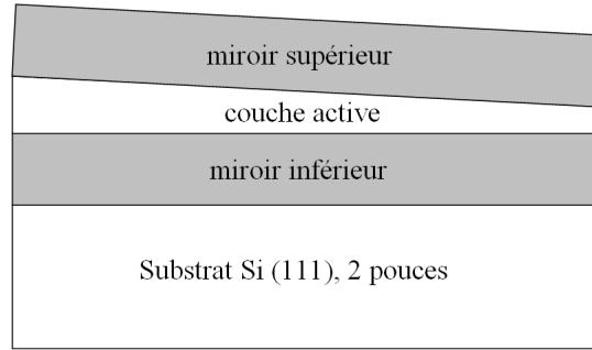
FIG. 2.18 – Représentation du gradient d'épaisseur de la couche active.
