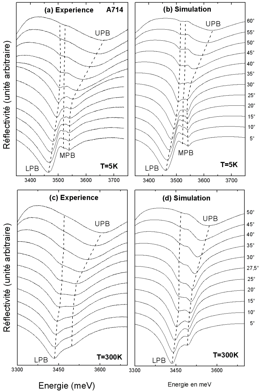
FIG. 3.5 – Les spectres de réflectivité en angle de l'échantillon A714 enregistrés à 5 K et à 300 K en polarisation TE sont comparés aux simulations utilisant les matrices de transfert.
