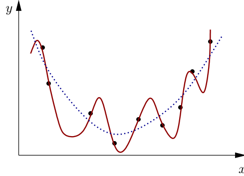
FIG. 2.4: Illustration du surapprentissage d'un modèle paramétrique. Lorsque le modèle est trop complexe, l'erreur empirique est faible sur la base d'apprentissage mais les fluctuations entre les exemples de la base d'apprentissage augmente l'erreur sur de nouvelles données.
