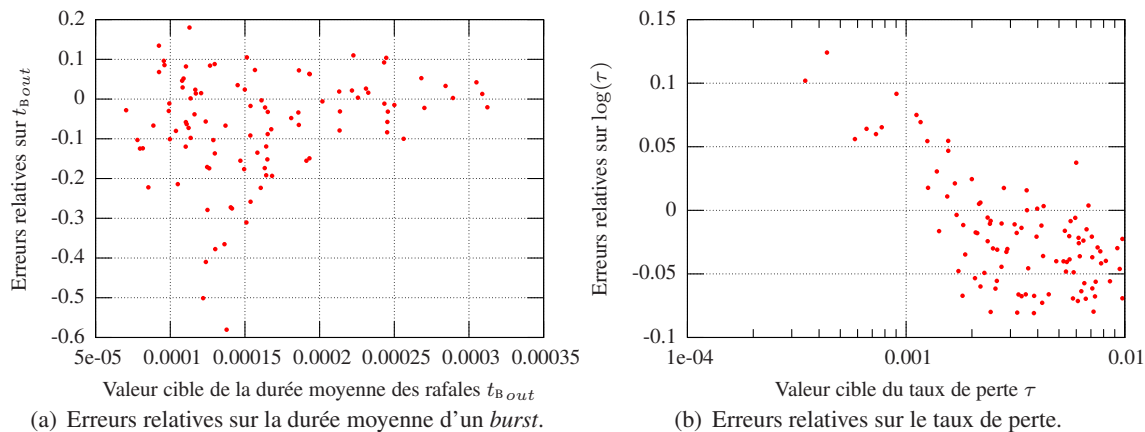
FIG. 5.10: Erreurs relatives commises par le réseaux de neurones pour la troisième file d'attente, les entrées du MLP étant calculées à partir des estimations des MLP amonts.
