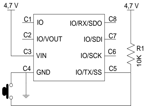
Gambar 3.5. Rangkaian IQRF
