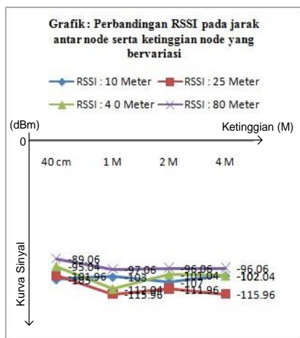
Gambar 4.5 Grafik perbandingan pengujian indoor untuk berbagai macam jarak
