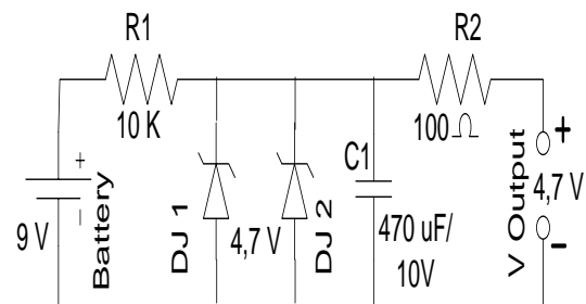
Gambar 3.3. Rangkaian catu daya
