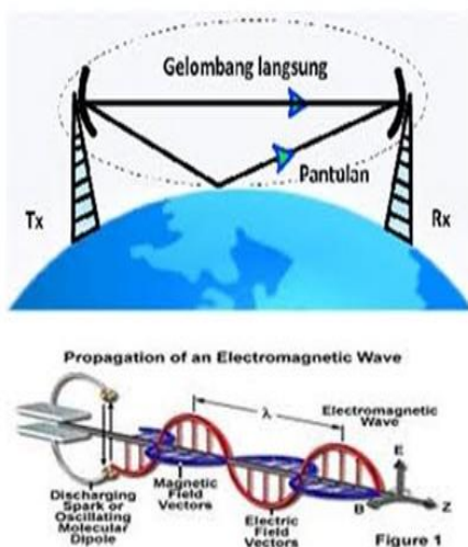
Gambar 2.1. Propagasi gelombang radio
