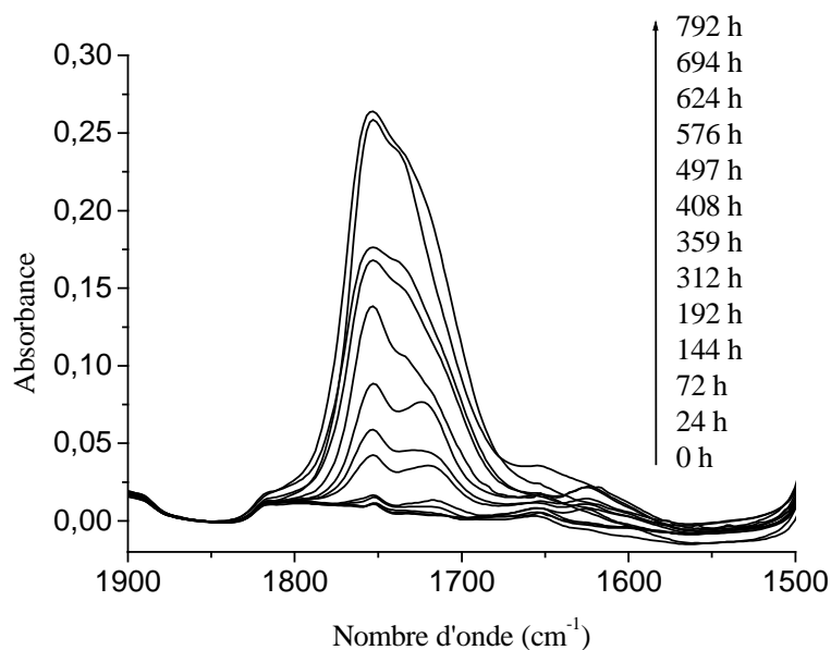
Figure 31 : Spectres IR de dépôts d'une solution aqueuse de PEO à \text{pH} = 3,1 au cours de la thermooxydation, [\text{PEO}] = 50 \text{ mg mL}^{-1} .
