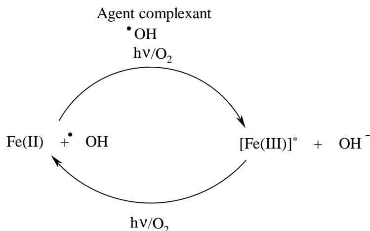
Figure 23 : Schéma de l'équilibre photostationnaire entre Fe(III) et Fe(II) en présence de composés organiques, [Fe(III)] représente toutes les formes de fer ferrique au cours du cycle [\text{Fe(II)}]/[\text{Fe(III)}] .
