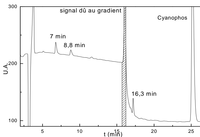
Figure A-62 : Chromatogramme ( \lambda_{\text{détection}} = 233 \text{ nm} ) d'une solution de cyanophos ( 8 \times 10^{-5} \text{ M} , \text{pH} = 5.5 ). Pic hachuré = signal dû au gradient.
