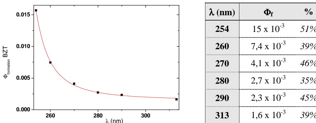
Figure A-32 : Effet de la longueur d'onde sur le rendement quantique de formation de BZT et évolution du pourcentage de formation.
