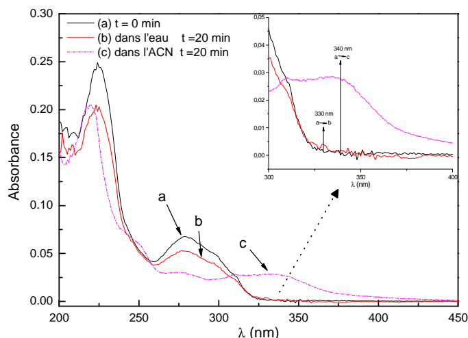
Figure A-45 : Evolution du spectre d'absorption de BZT ( C_o = 1,2 \times 10^{-5} \text{ mol.L}^{-1} , pH = 5,7), milieu aéré, \lambda_{excitation} = 310 \text{ nm} . (a) en solution aqueuse (eau ou ACN) non irradiée, (b) irradié 20 minutes dans l'eau, (c) irradié 20 min en solution dans l'Acétonitrile (ACN).
