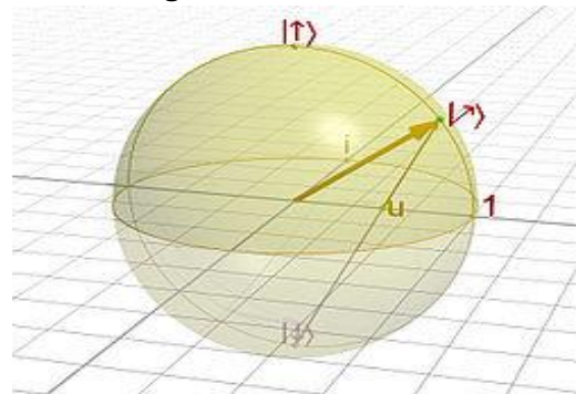
Figura 6. Esfera de Bloch
