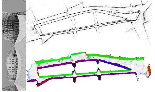
FIG. 5 – A gauche : image de la scène synthétique. A droite : résultats de SfM et la surface finalement estimée.
