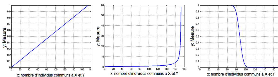
FIGURE 2.7: Différents comportements d'une mesure d'intérêt m (linéaire, concave, convexe).
