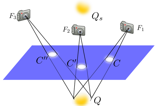
FIGURE 2 – Schéma illustrant l'ensemble de notre méthode. La lumière (modélisée par une quadrique Q_s ) laisse plusieurs traces spéculaires sur le plan sous forme de coniques ( C, C', C'' ). Nous approximations ces spécularités par des coniques ( C, C', C'' ). La quadrique Q correspond à la symétrique de la quadrique Q_s par rapport au plan de la scène.
