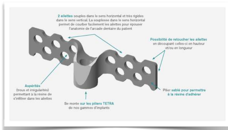
Figure 3: « Pilier-bar » EUROTECHNIZATM®
