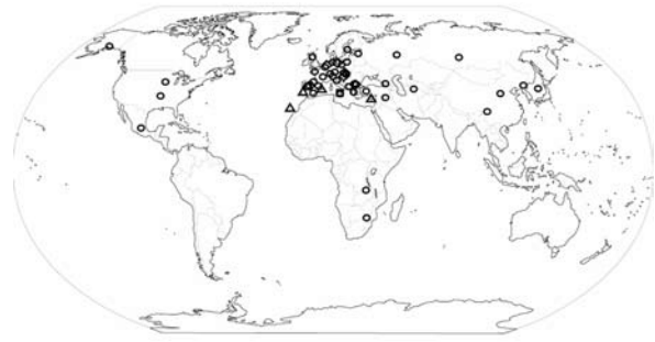
Fig. 294. World distribution map of Gomphonema rosenstockianum (triangle), G. tergestinum (circle), G. angustius (square), G. supertergestinum (diamond).
