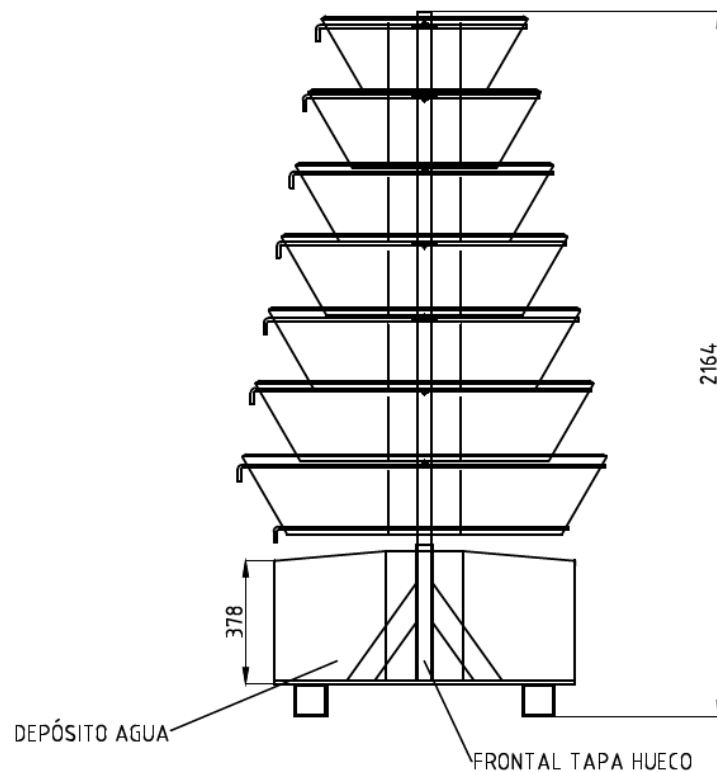
Figura 1. Estructura metálica con bandejas de cultivo en altura
