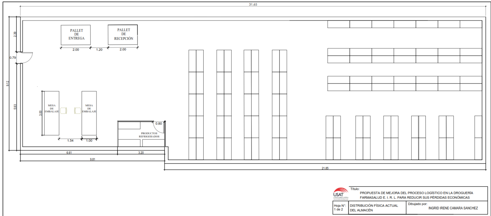
Figura 10. Distribución física actual del almacén de la Droguería Farmasalud E. I. R. L.
