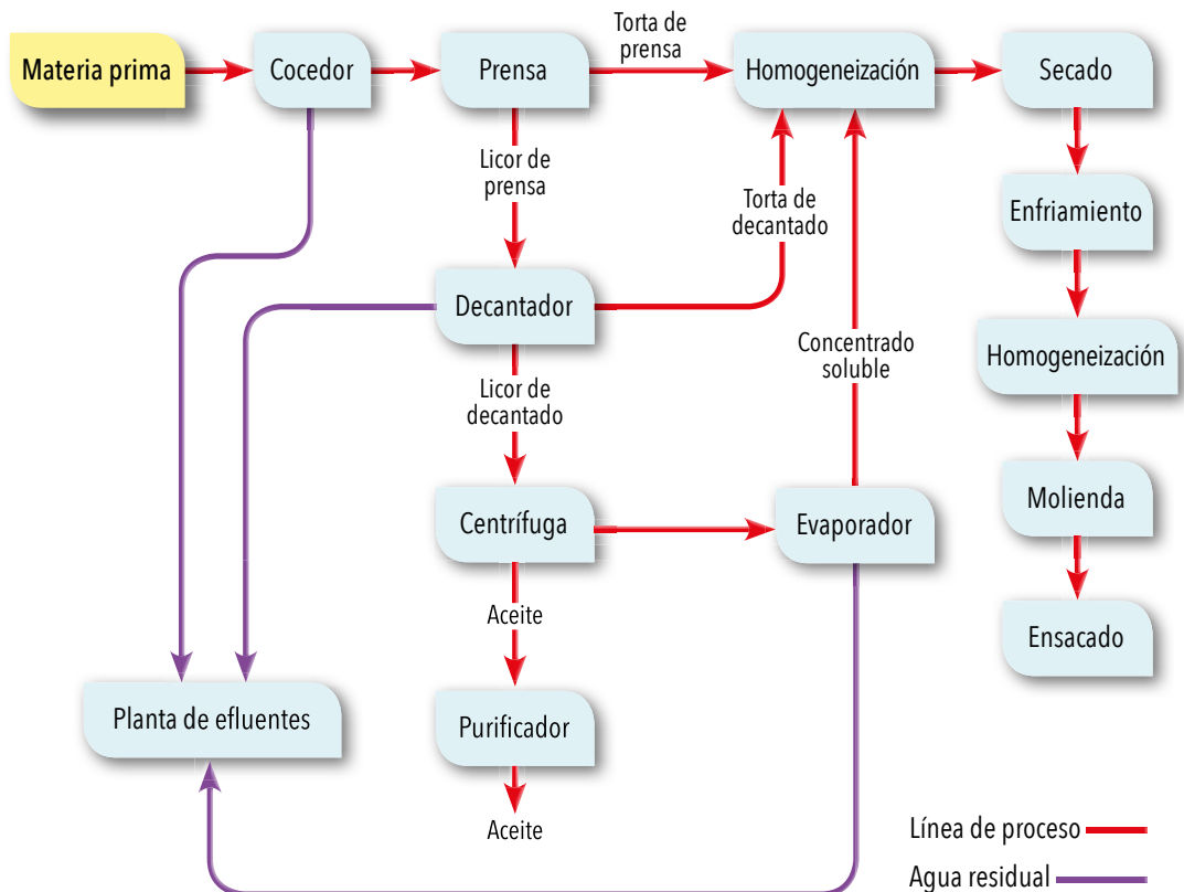
Figura 5. Proceso de producción de harinas y aceites de pescado [3].
