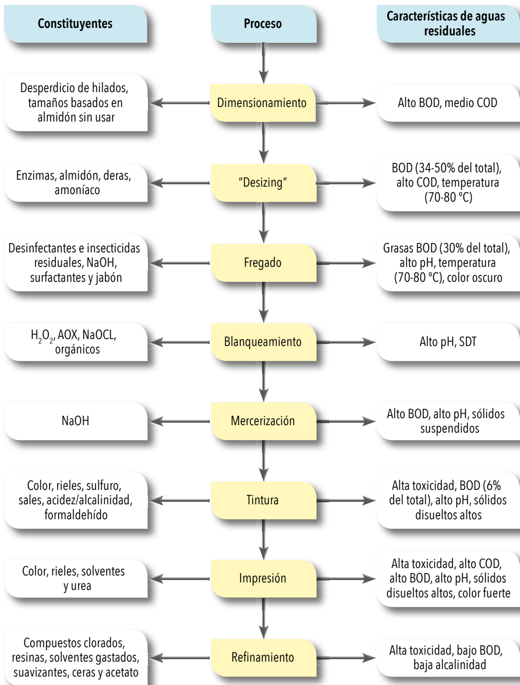
Figura 5. Componentes dos principais poluentes envolvidos nas várias etapas do processamento húmido da indústria têxtil [21].
