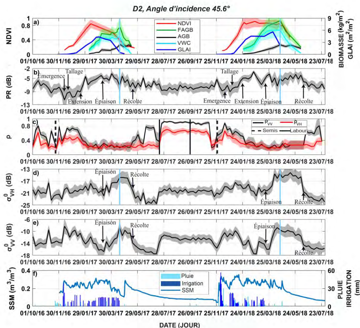
Figure III. 10 : Séries temporelles de PR , \sigma_{VV}^0 , \sigma_{VH}^0 , \rho_{VV} et \rho_{VH} à 45.6^\circ d'incidence sur D2 et pendant deux saisons agricoles 2016–2017 et 2017–2018. Le NDVI, le LAI mesuré, le VWC mesuré, la FAGB et l'AGB sont tracés dans le premier subplot. Les valeurs moyennes sont représentées par des lignes continues et les écarts types par les zones remplies entourant les courbes. Les précipitations, l'irrigation et le SSM sont tracés dans le dernier subplot. Les stades phénologiques du blé et les événements de travail du sol sont superposés. La chute du VWC à la fin de la saison est représentée par une ligne verticale bleue sur les séries temporelles du rapport de polarisation et des coefficients de rétrodiffusion.
