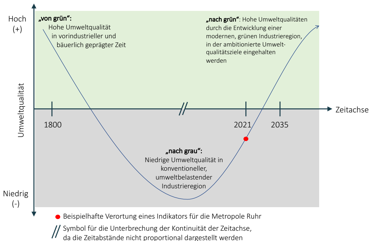
Abbildung 1-1: Prinzipdarstellung mit beispielhafter Verortung eines Umweltindikators für die Metropole Ruhr auf einer grundsätzlichen, skizzenhaften Entwicklungslinie der Umweltqualität „von grün nach grau nach grün“
