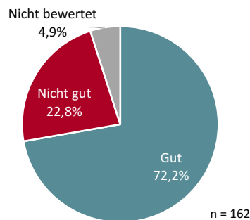
Abbildung 4-11: Chemischer Zustand 75 der Fließgewässer Emscher, Lippe und Ruhr einschließlich ihrer Nebenflüsse/Bäche
