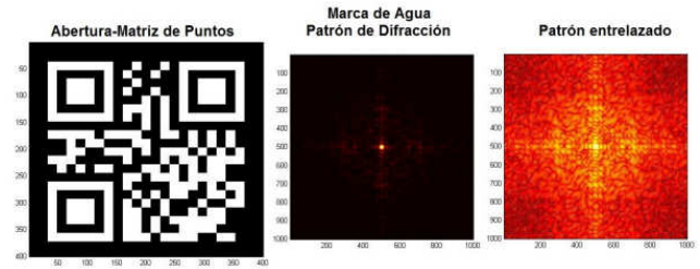
Figure 8. Abertura – Marca de Agua – Patrón entrelazado del texto-cifrado: INAOE---
