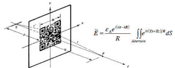
Figura 6. Sistema de la propagación sobre las rejillas para la obtención de los patrones de difracción.
