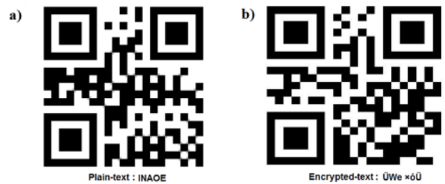
Figure 9. Códigos QR con a) texto plano: INAOE y b) su texto cifrado DES.
