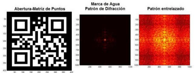
Figure 10. Abertura – Marca de Agua – Patrón entrelazado del texto-cifrado: Alejndro.
