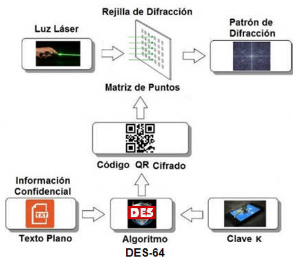
Figura 1. Esquema de inserción de la marca de agua para la generación de un patrón de difracción.
