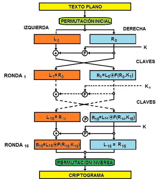
Figura 3. Cálculo de cifrado en el algoritmo DES.
