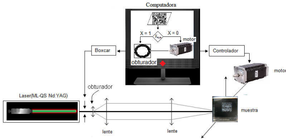
Figura 10. Sistema de daño óptico automatizado.
