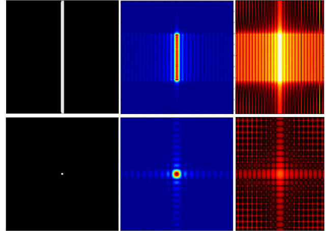
Figura 8. Ejemplos de patrones de radiación, rejilla-patrón-entrelazado.
