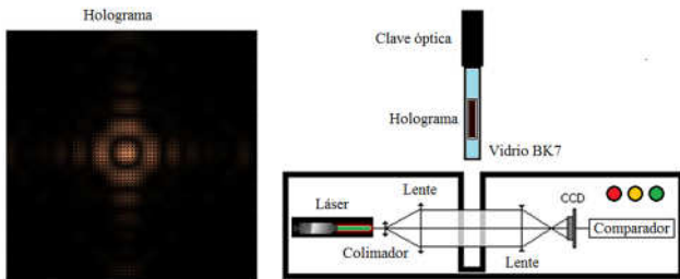
Figura 11. Sistema de lectura de la clave óptica.
