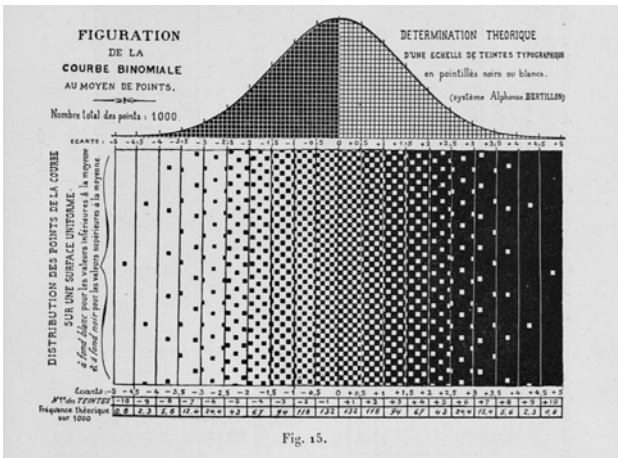
Abbildung 31: »Figuration de la courbe binomiale«: Bertillons Markierung des sozialen Raumes. Quelle: Bertillon und Chervin 1909, S. 61.
